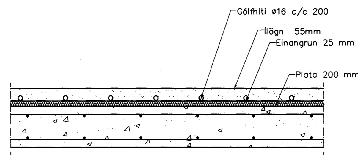
Gólfhit. Sníð í milliþötu, 1:10
