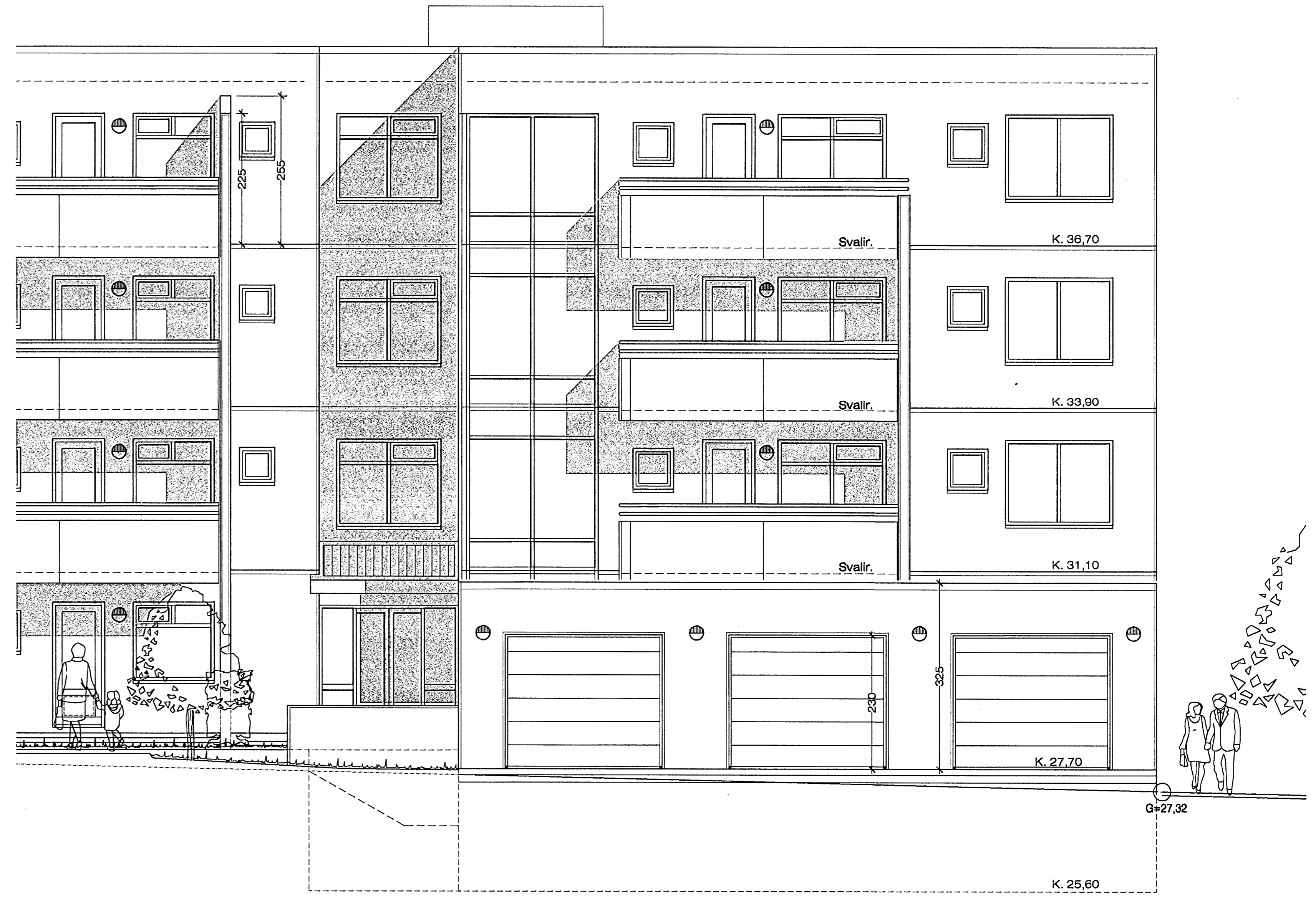
Séð framaná - Bilageymslur. 1 : 50
