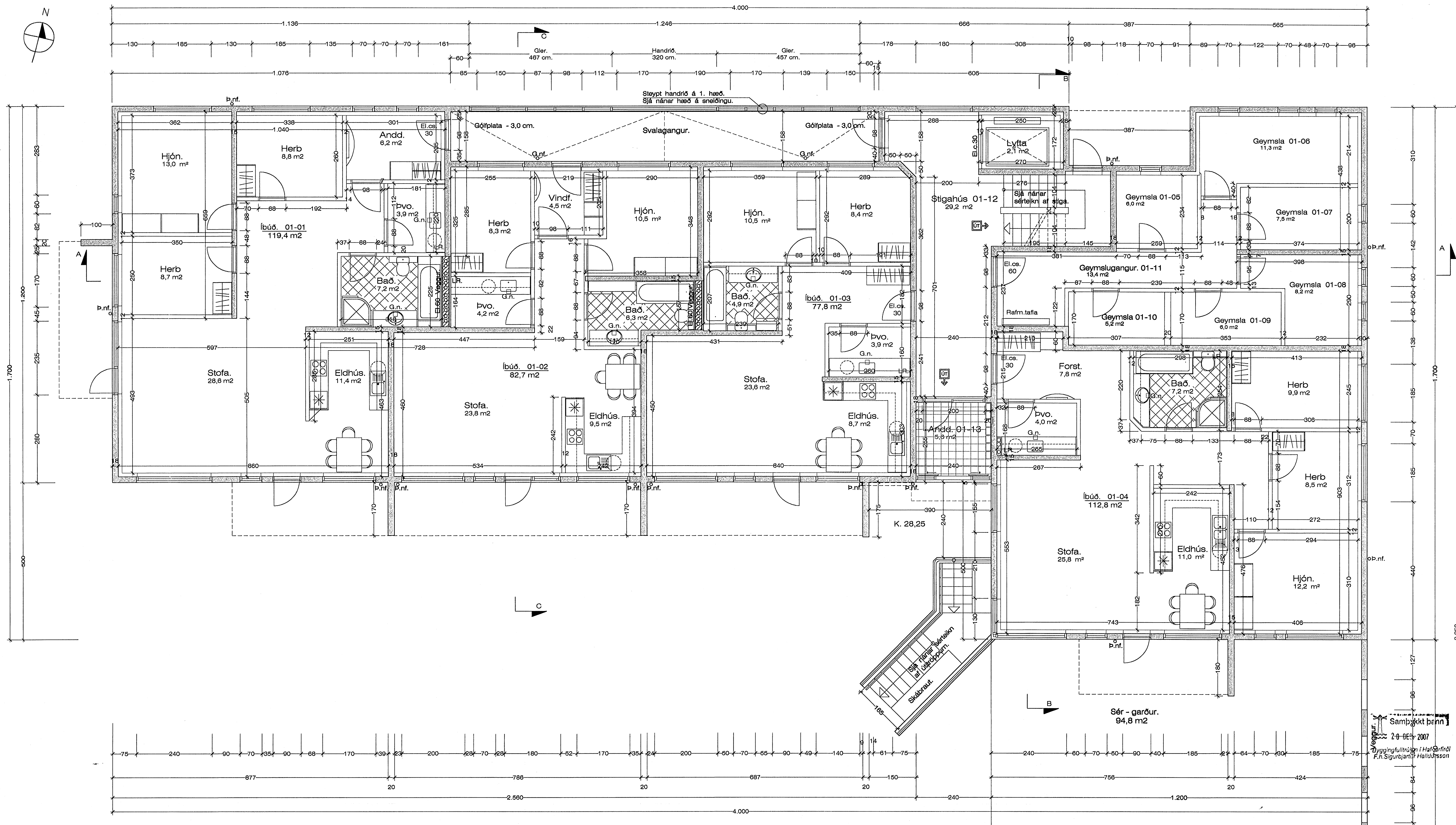
Grunnmynd Jarðhæðar. 1 : 50
