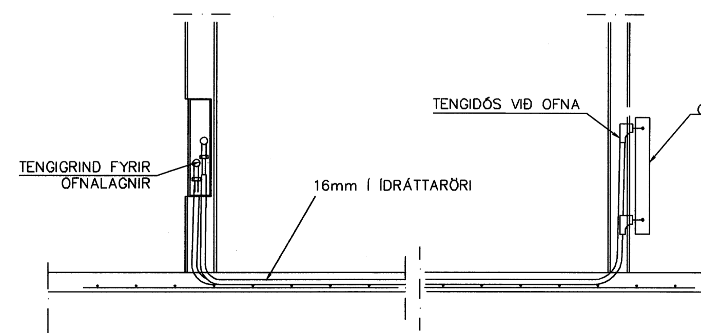
TENGING OFNALAGNALAGNA 1:20
