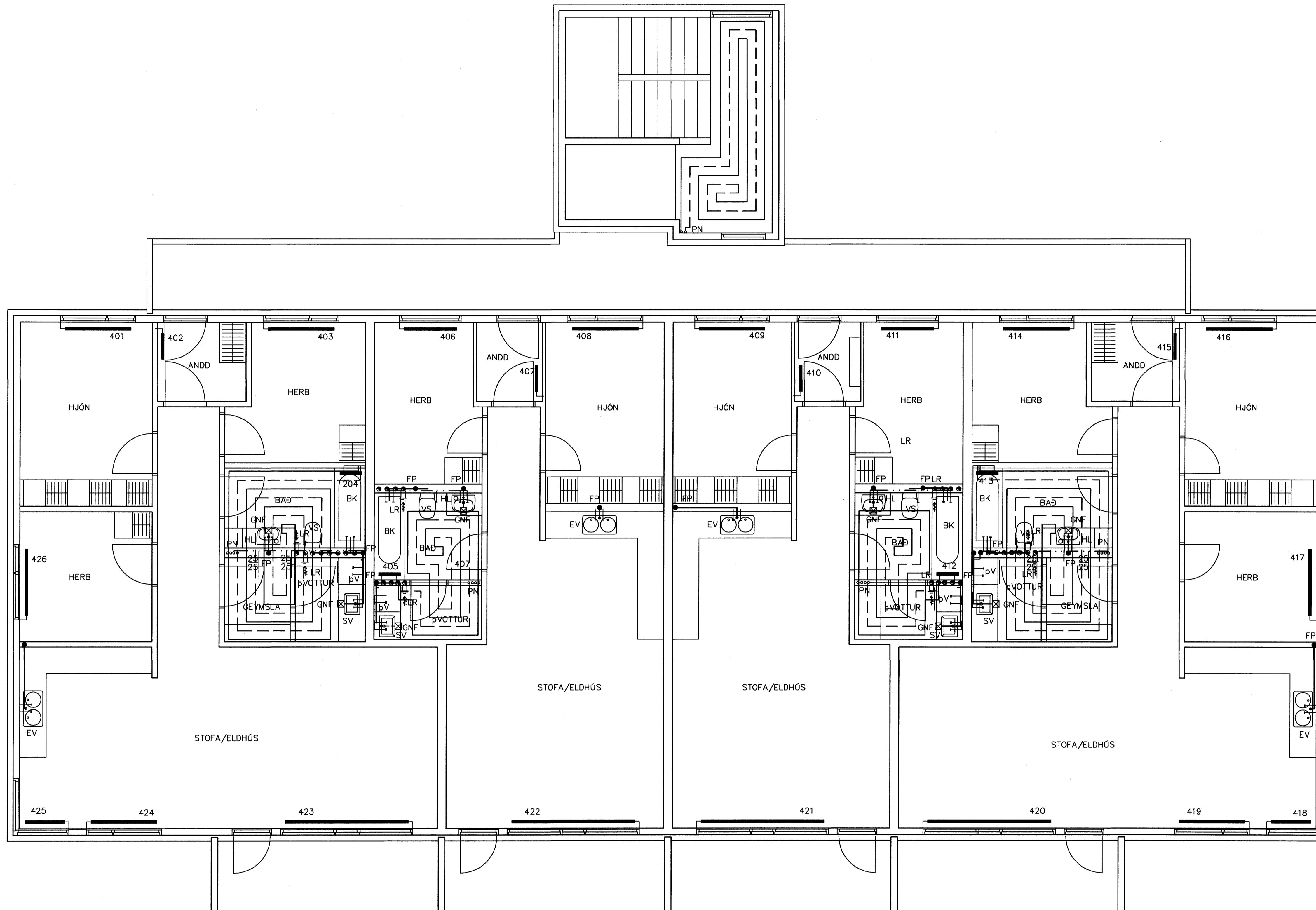
GRUNNMYND 4 HÆÐAR 1:50
