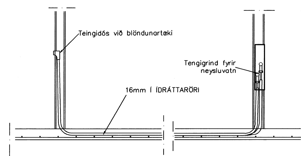
TENGING NEYSLUVATNSLAGNA 1:20
