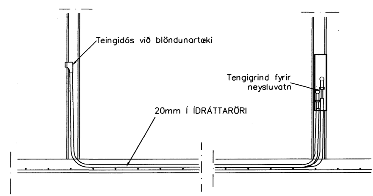
TENGING NEYSLUVATNSLAGNA 1:20
