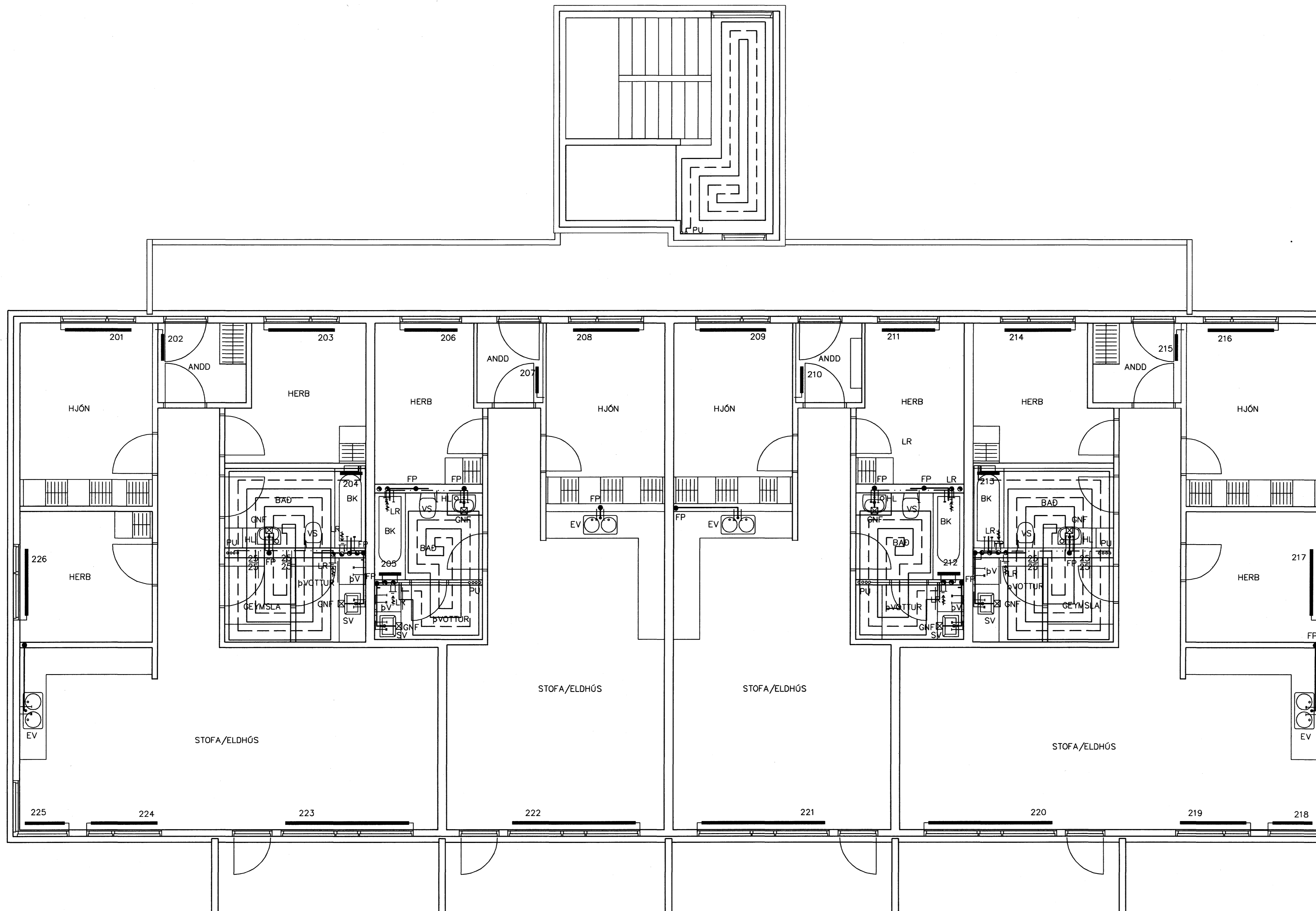
GRUNNMYND 2 HÆÐAR 1:50
