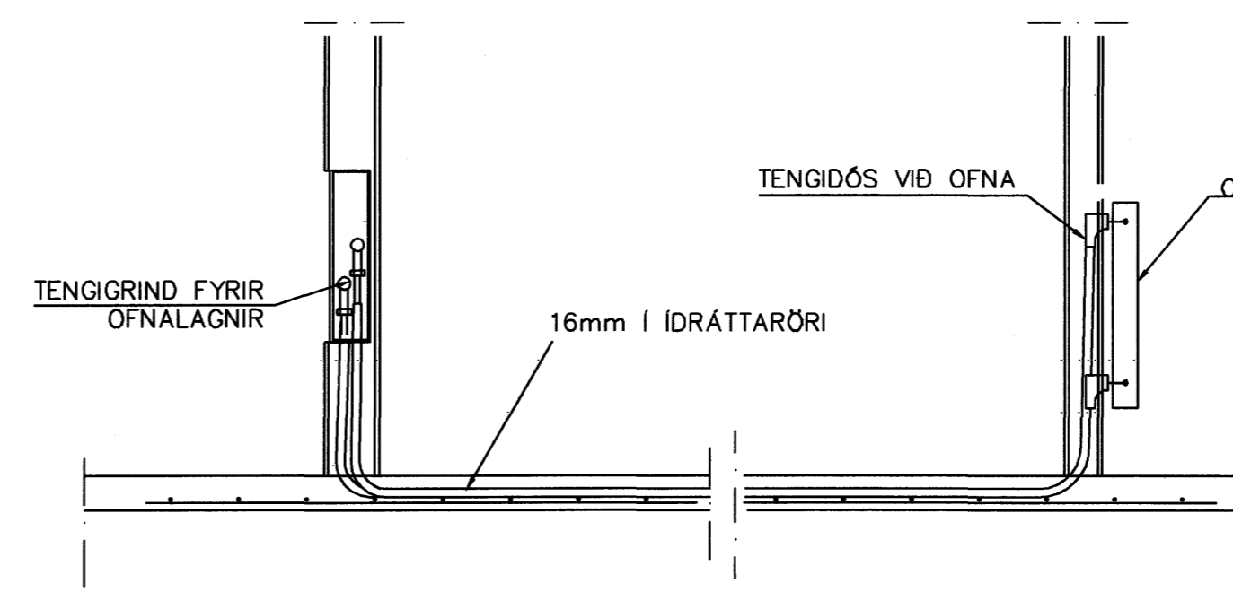
TENGING OFNALAGNALAGNA 1:20
