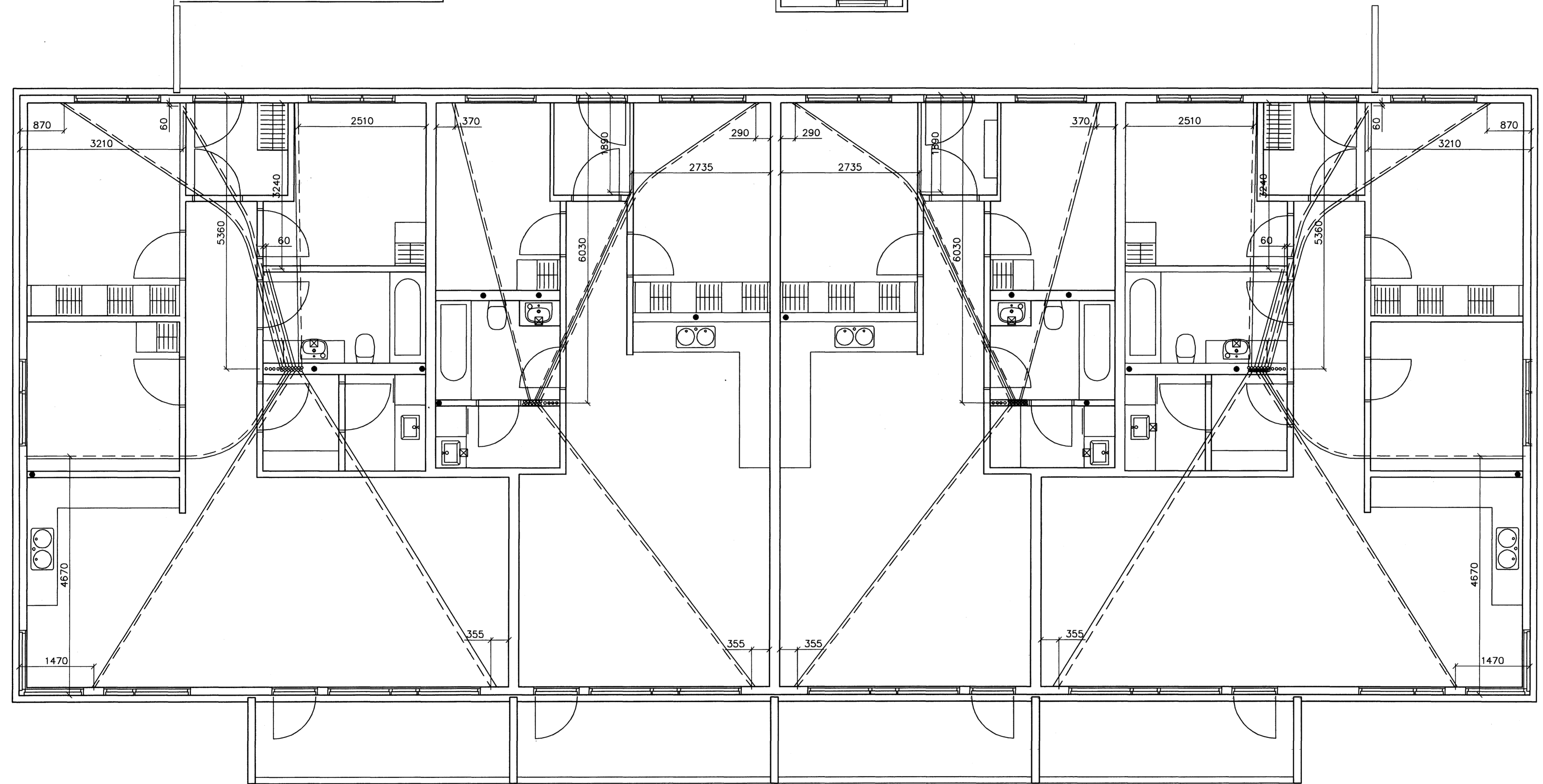
GRUNNMYND 4 HÆÐAR 1:50
