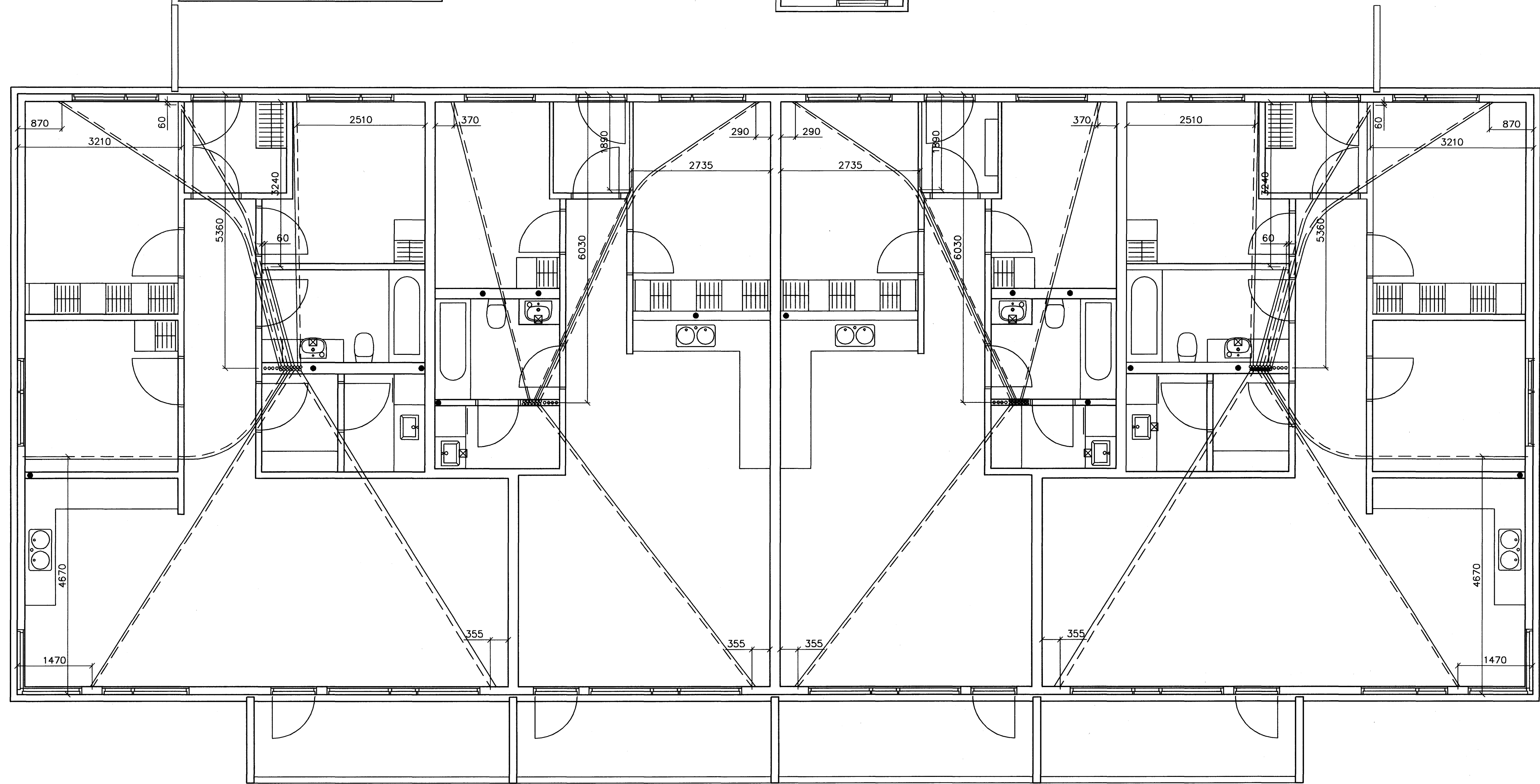
GRUNNMYND 2 HÆÐAR 1:50
