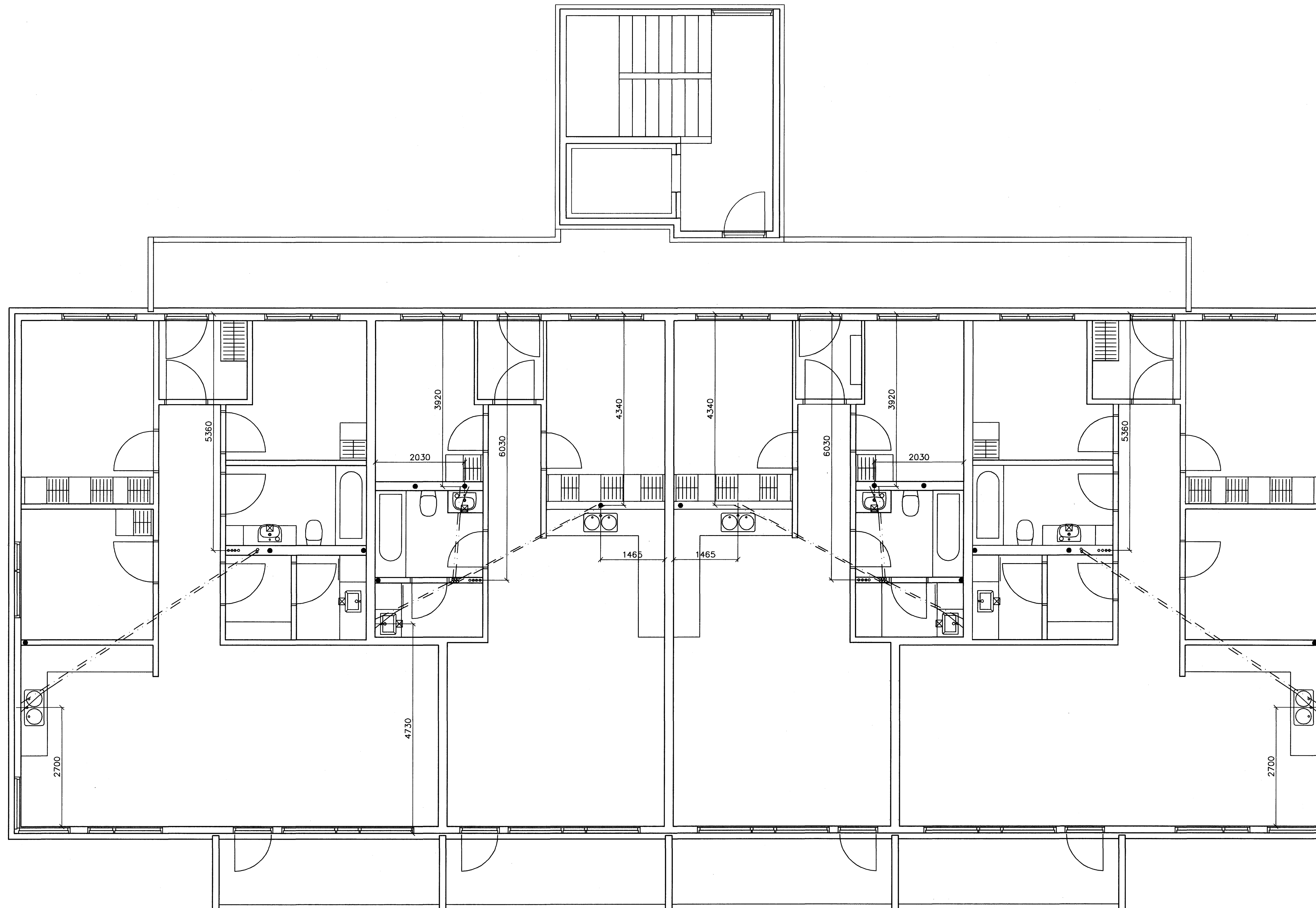
GRUNNMYND 3 HÆÐAR 1:50
