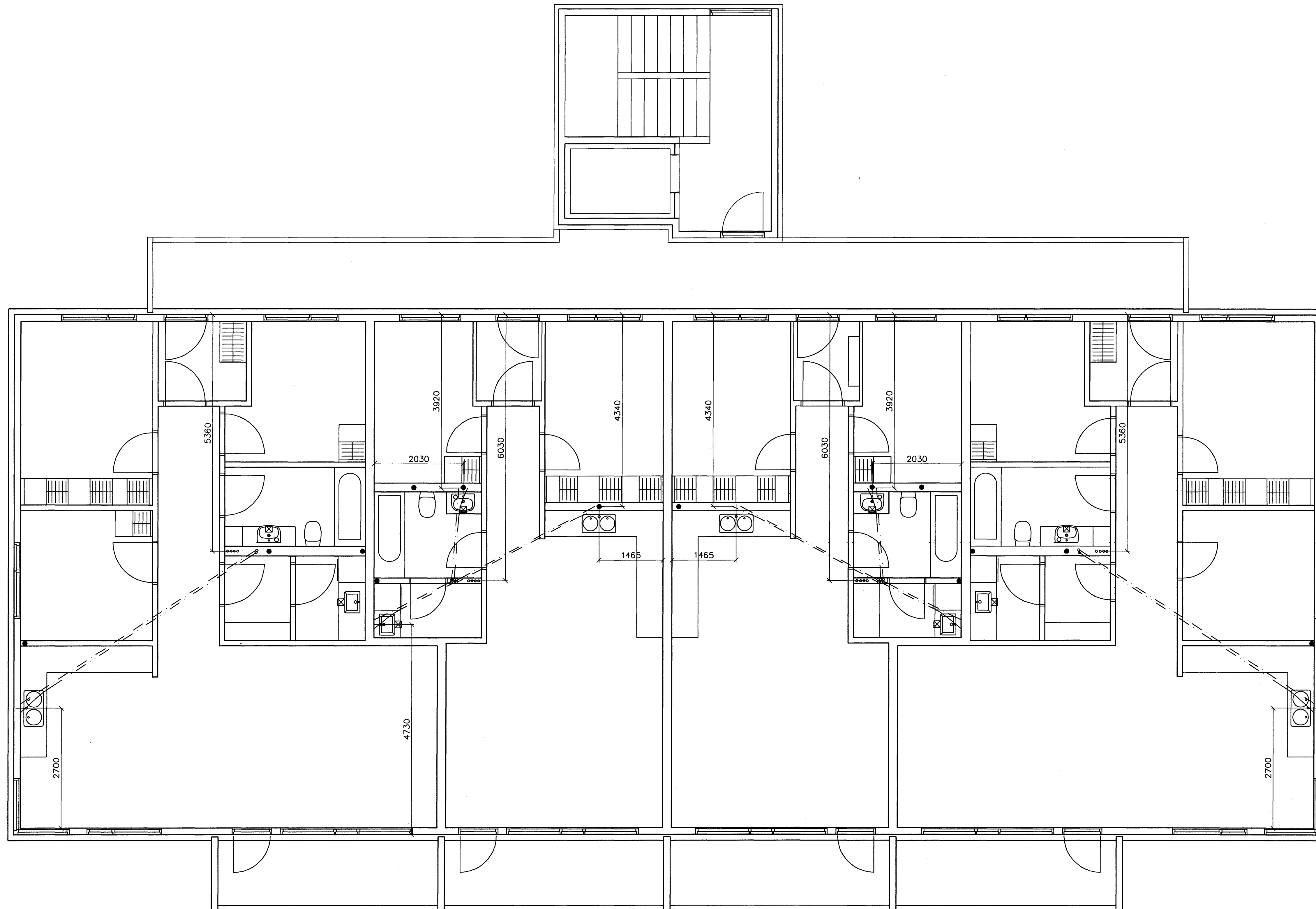
GRUNNMYND 2 HÆÐAR 1:50
