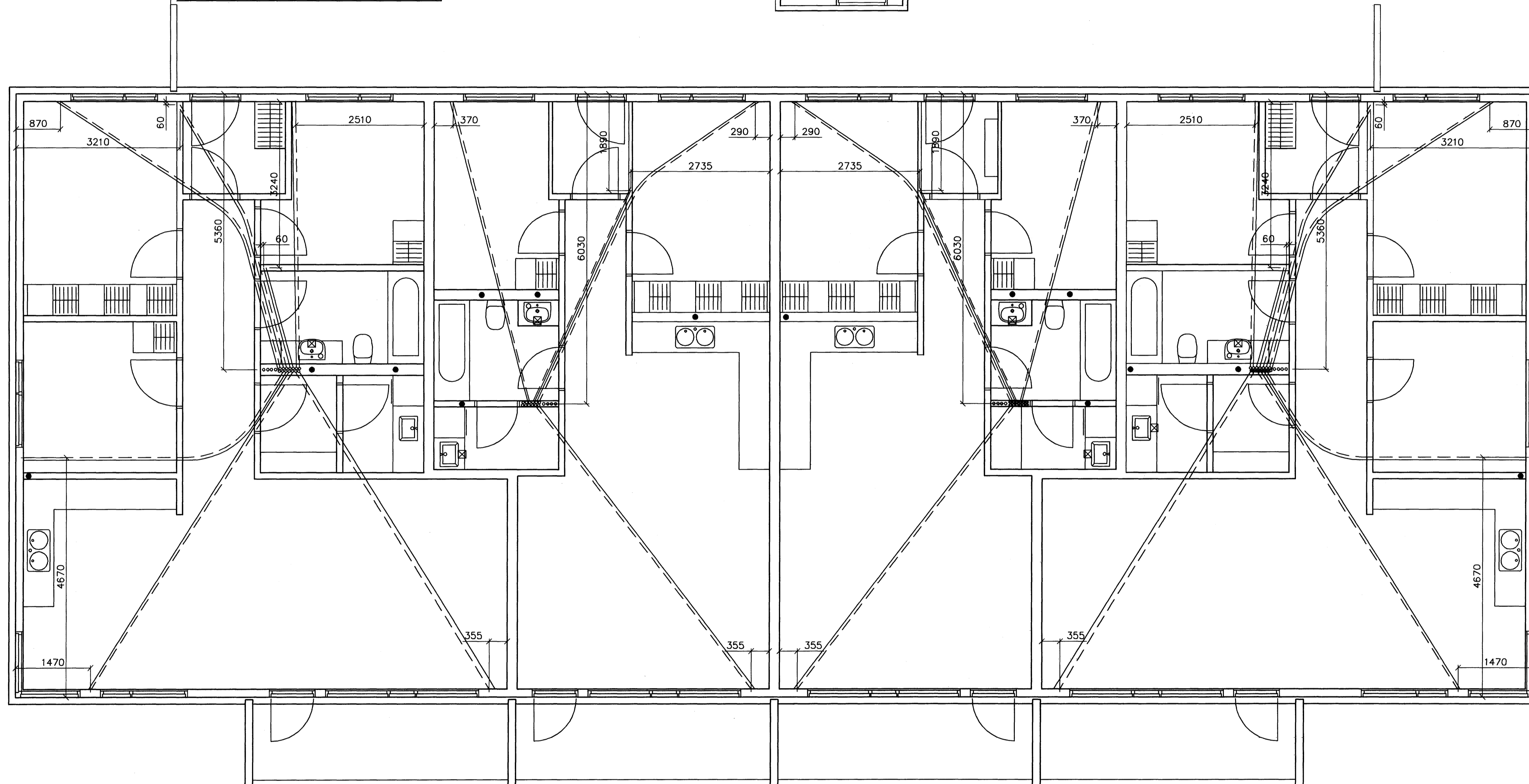
GRUNNMYND 1 HÆÐAR 1:50
