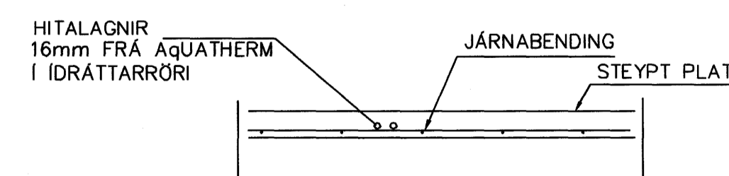
LAGNIR, SNIÐ, 1:20
