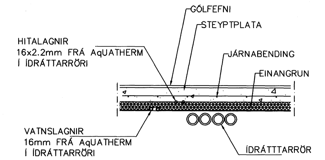
LAGNIR, SNIÐ, 1:20
