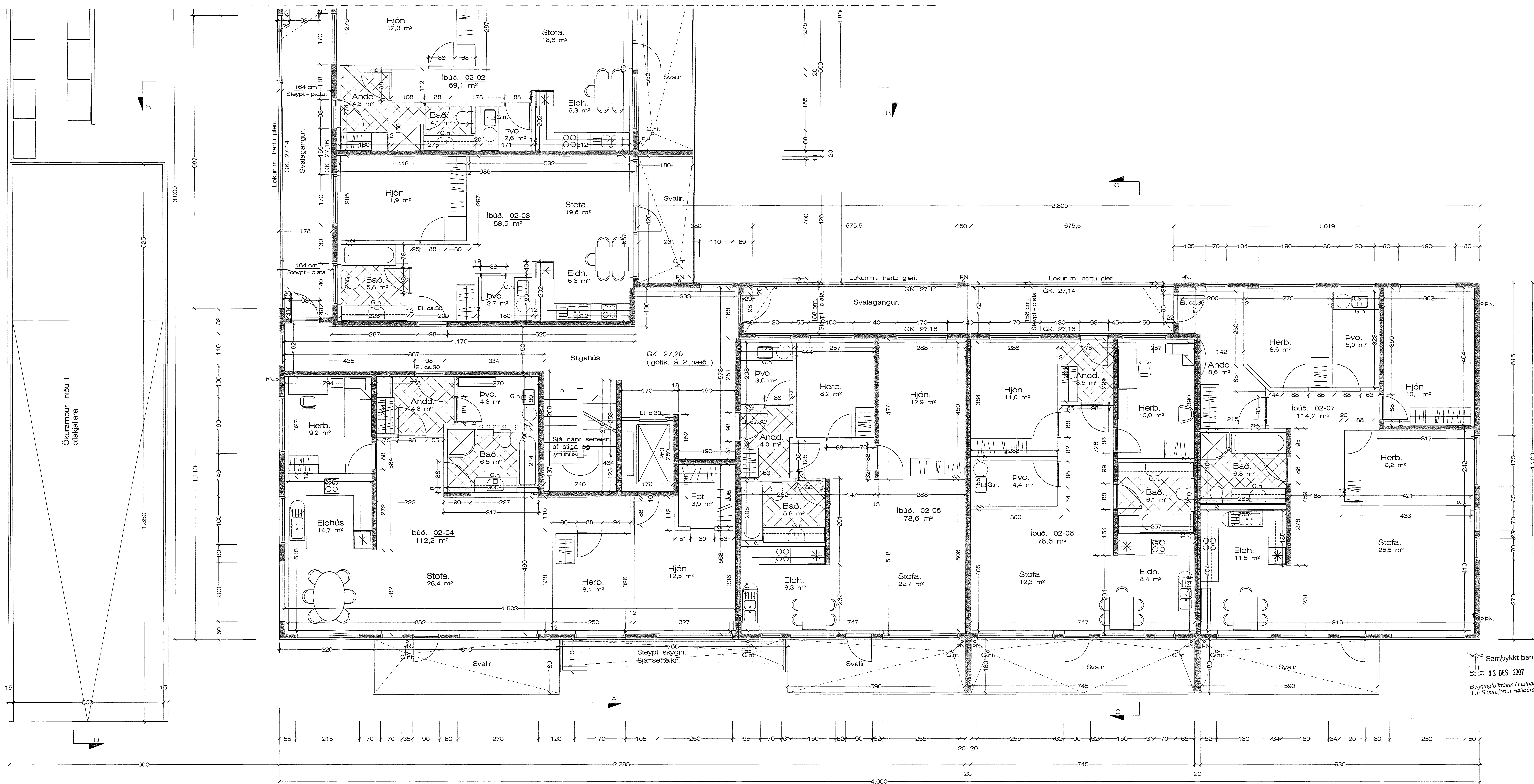
Grunnmynd 2. - 4. hæð. 1 : 50
