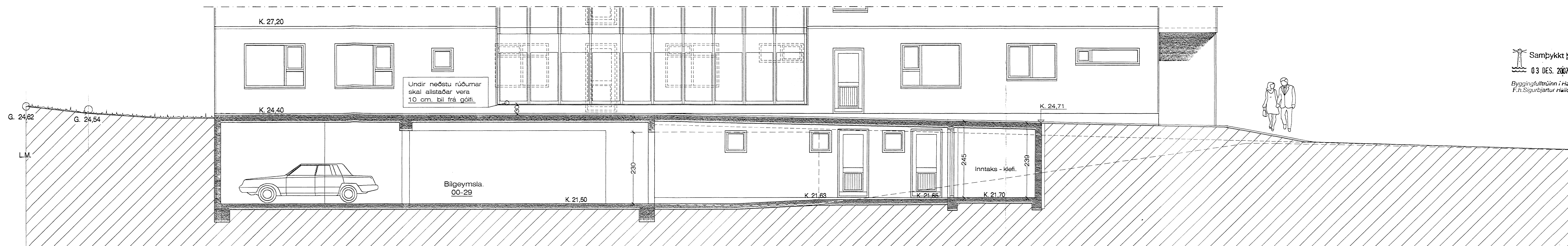
Sneiðing. D - D 1 : 50 Gegnum Inntaksklefa.
