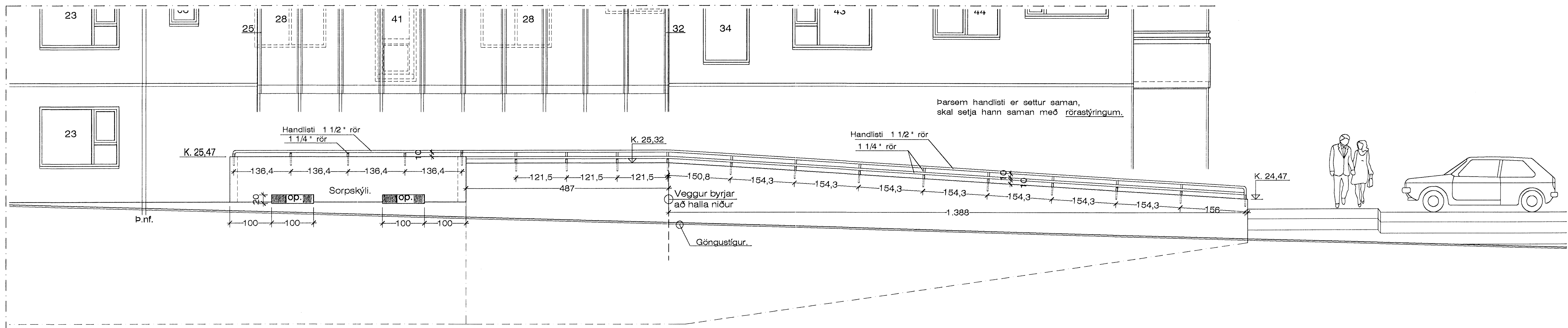
Handrið á stoðvegg við skábraut niður í bílgeymslu. Séð frá göngustígnum. 1:50
