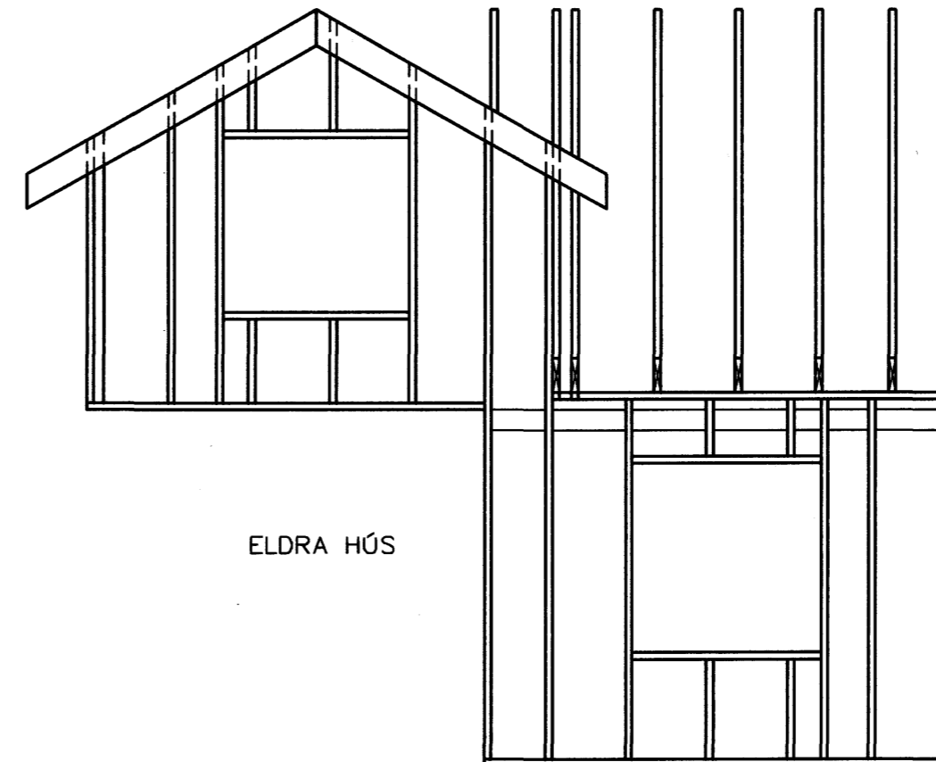
ÁSÝND VESTUR 1:50
