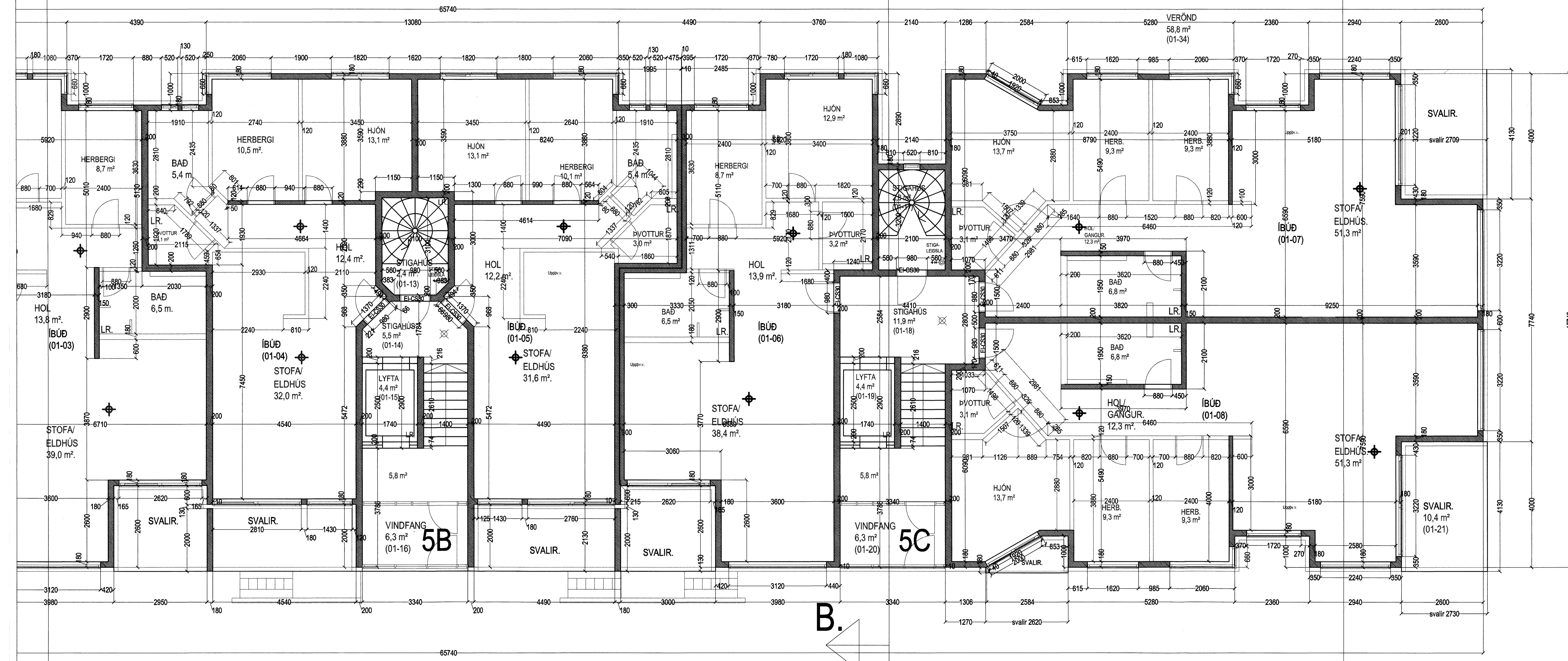
Grunnmynd 1 hæð. HÚS B og C. GRUNNMYND 1. HÆÐ. MKV. 1:50.
