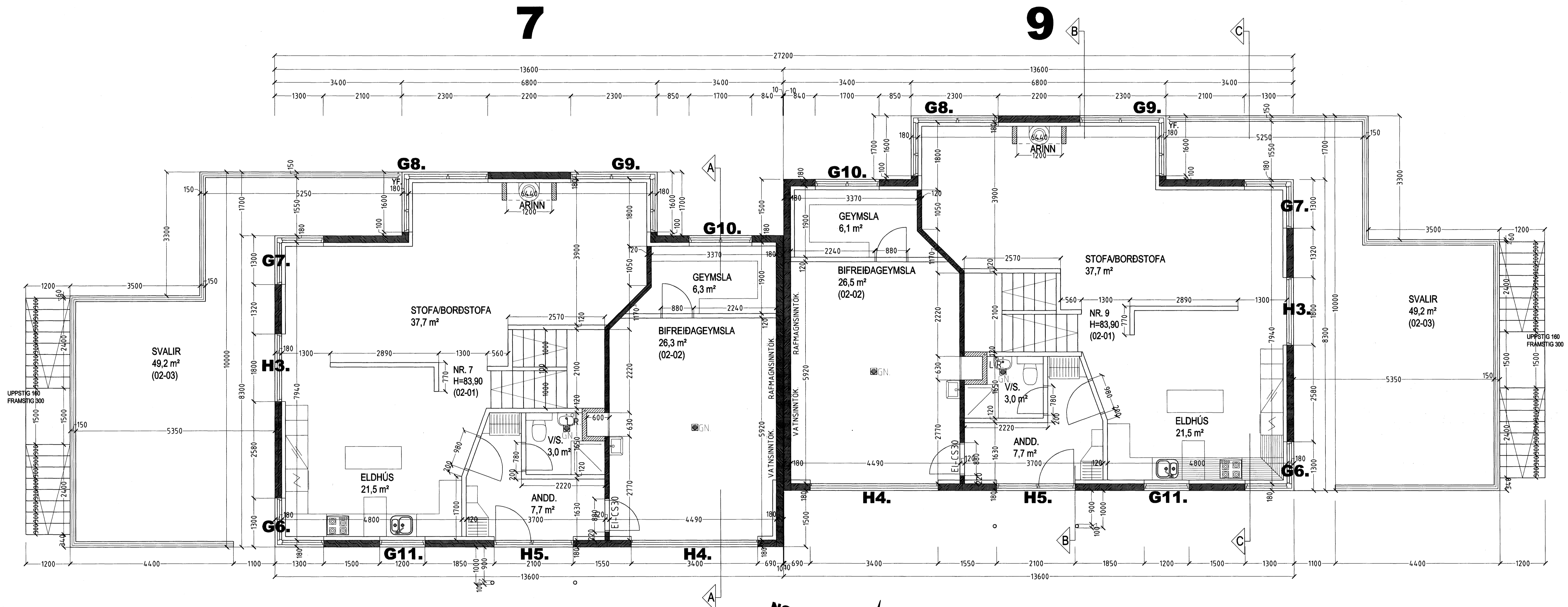
GRUNNMYND 2. HÆÐ MKV. 1:50.
