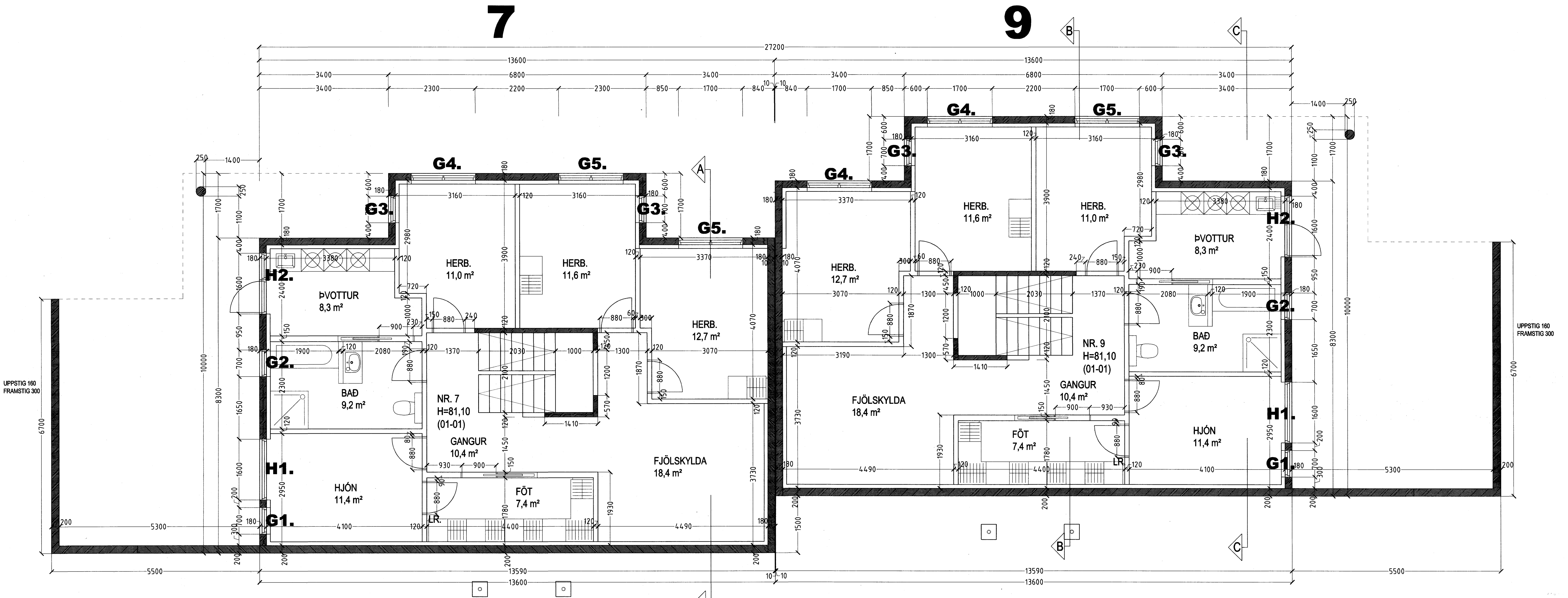
GRUNNMYND 1. HÆÐ MKV. 1:50.
