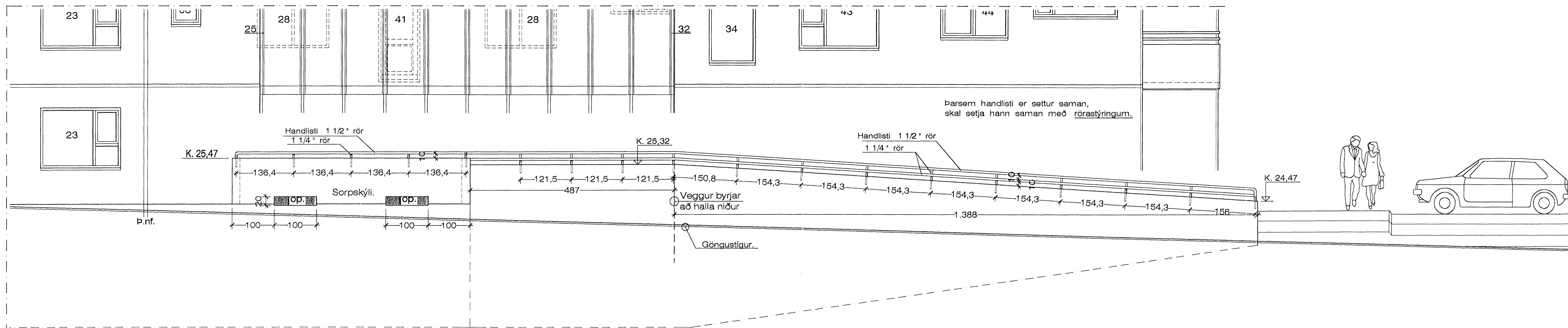
Handrið á stoðvegg við skábraut niður í bílgeymslu. Séð frá göngustígunum. 1:50
