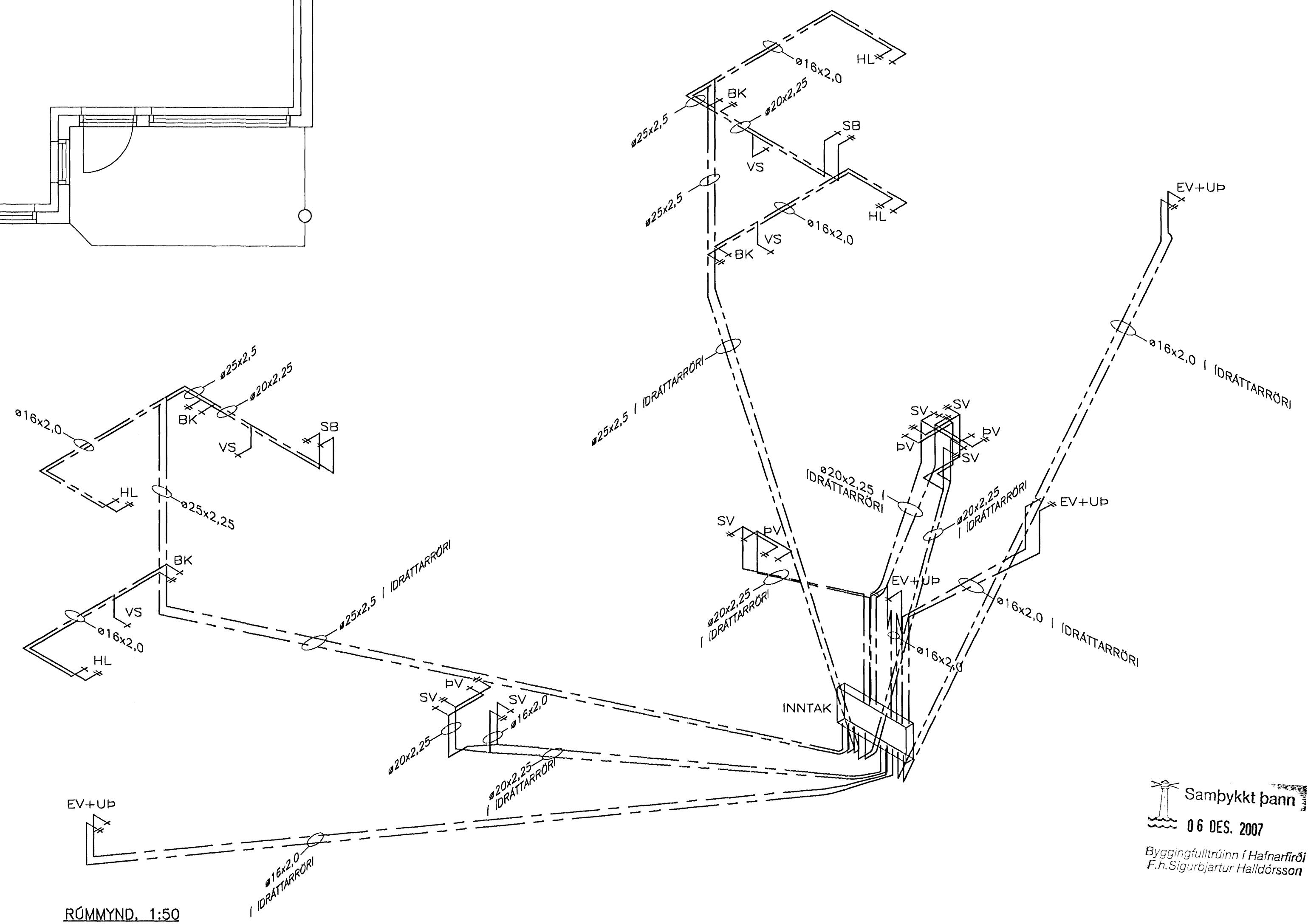
RÖMMYND. 1:50
