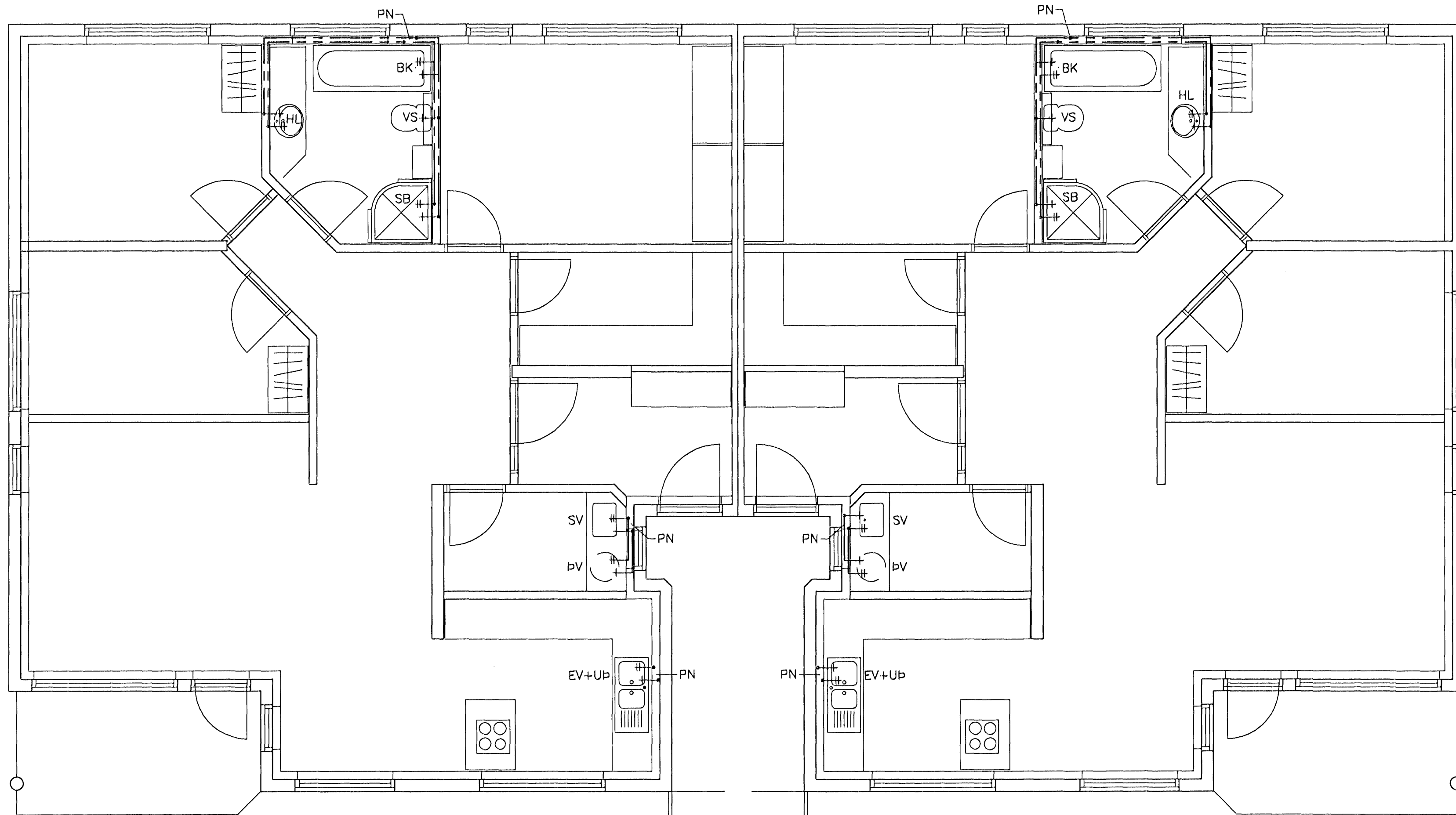
GRUNNMYND 2.HÆÐ. 1:50
