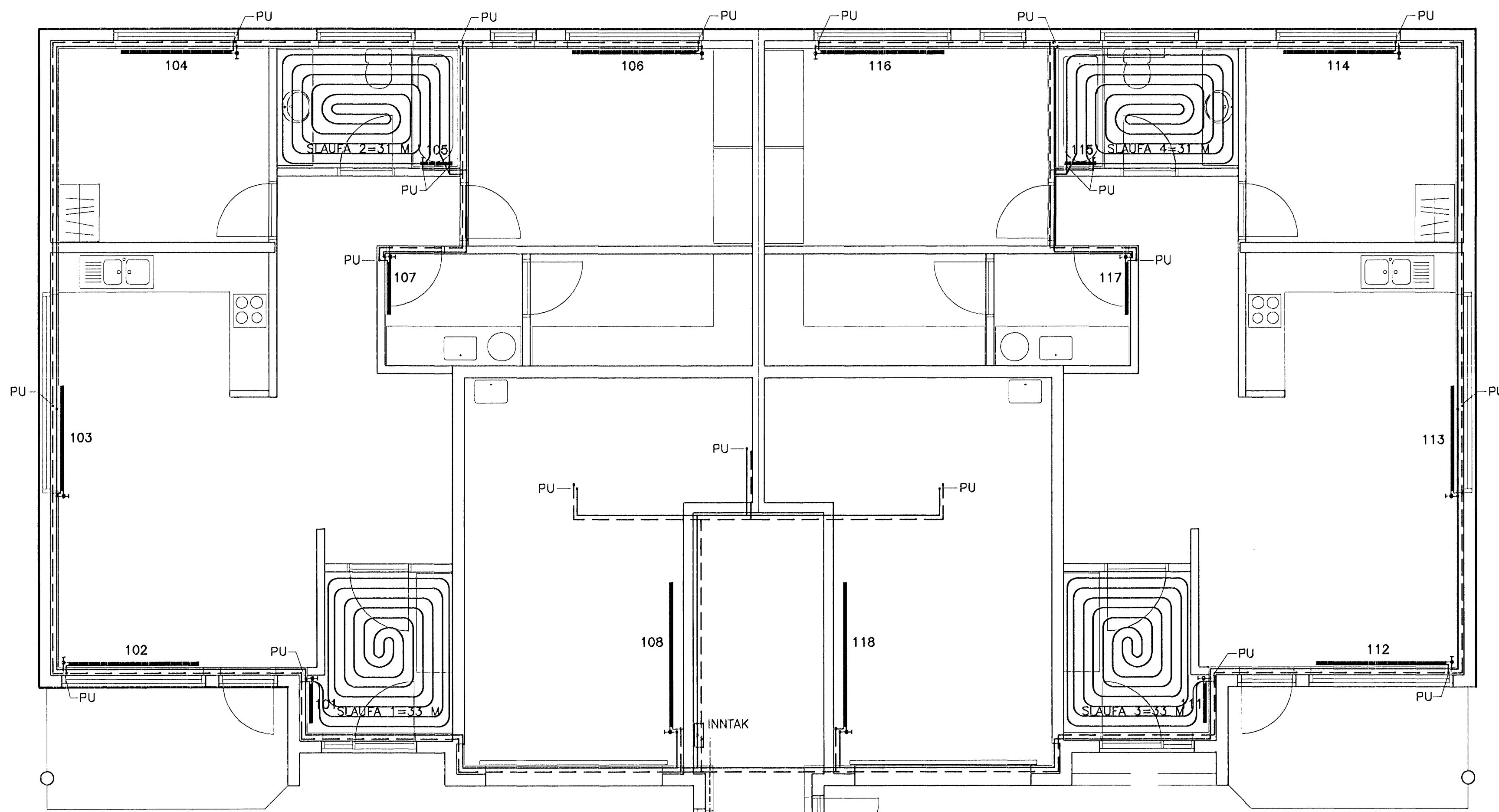
GRUNNMYND 1.HÆÐ
