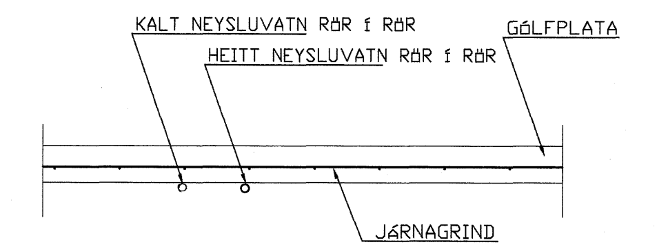
SNID Í GÖLFPLATU MED NEYSLUVATNI RÖR Í RÖR 1:20
