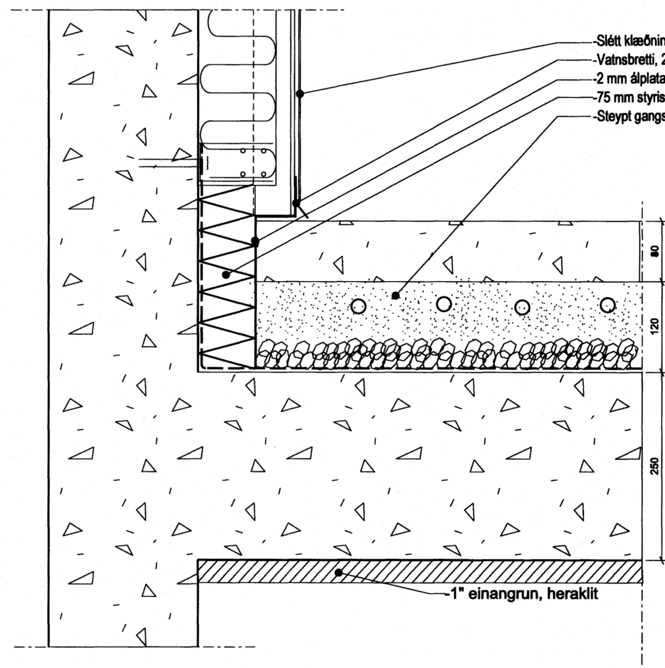
6 DEILI 1:5 Frágangur við plötu yfir kjallara
