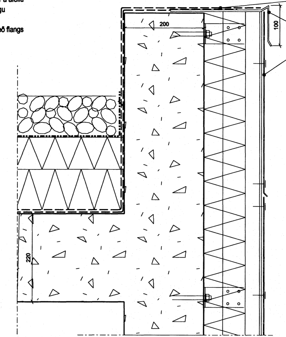
3 DEILI 1:5 Þakfrágangur, almennt, slétt klæðning
