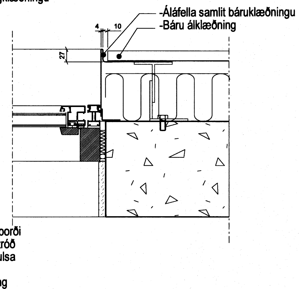
8 DEILI 1:5 Hliðarstykki glugga, báruálklæðning
