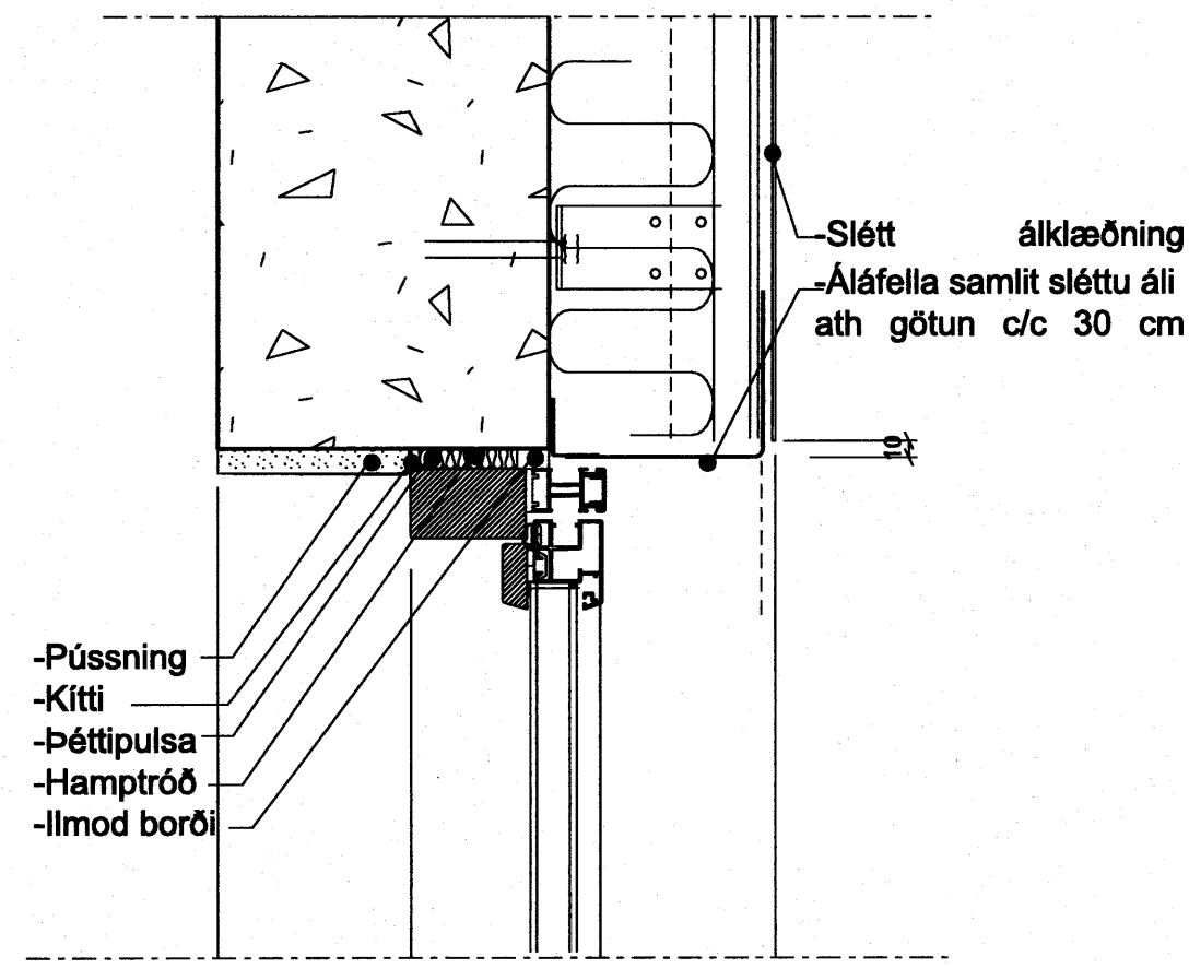
2 DEILI 1:5 Efri brún glugga, slétt álklaðning
