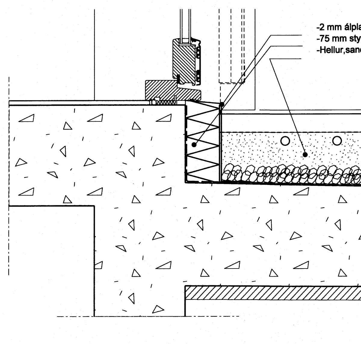
9 DEILI 1:5 Botnstykki útidyrarúða á jarðhæð
