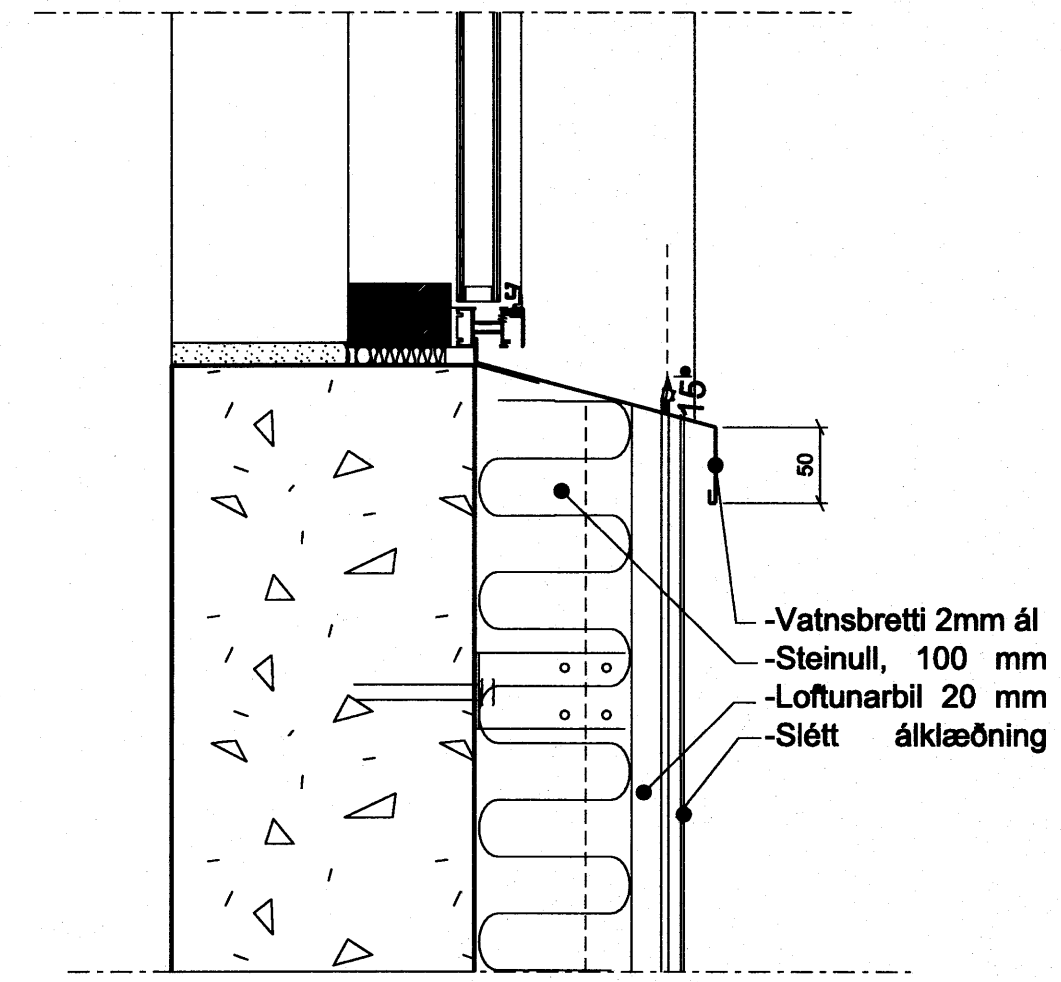
4 DEILI 1:5 Neðri brún glugga, slétt álklaðning
