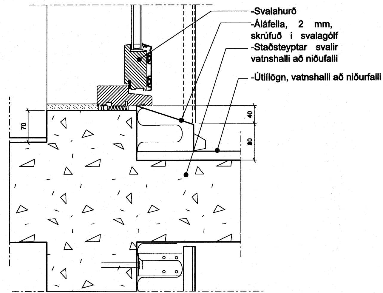
6 DEILI 1:5 Botnstykki svaladyra
