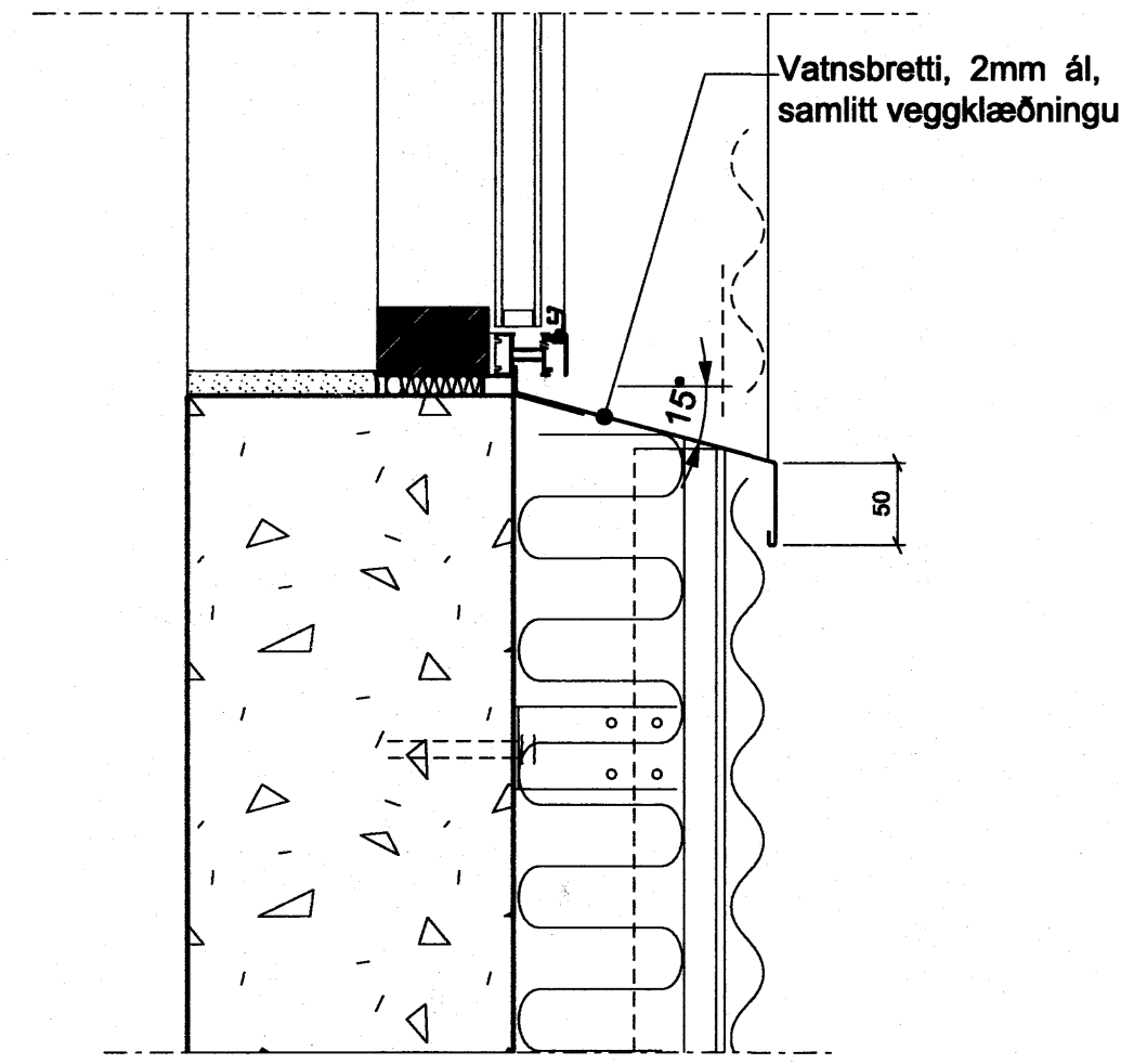
3 DEILI 1:5 Neðri brún glugga, báruklæðning
