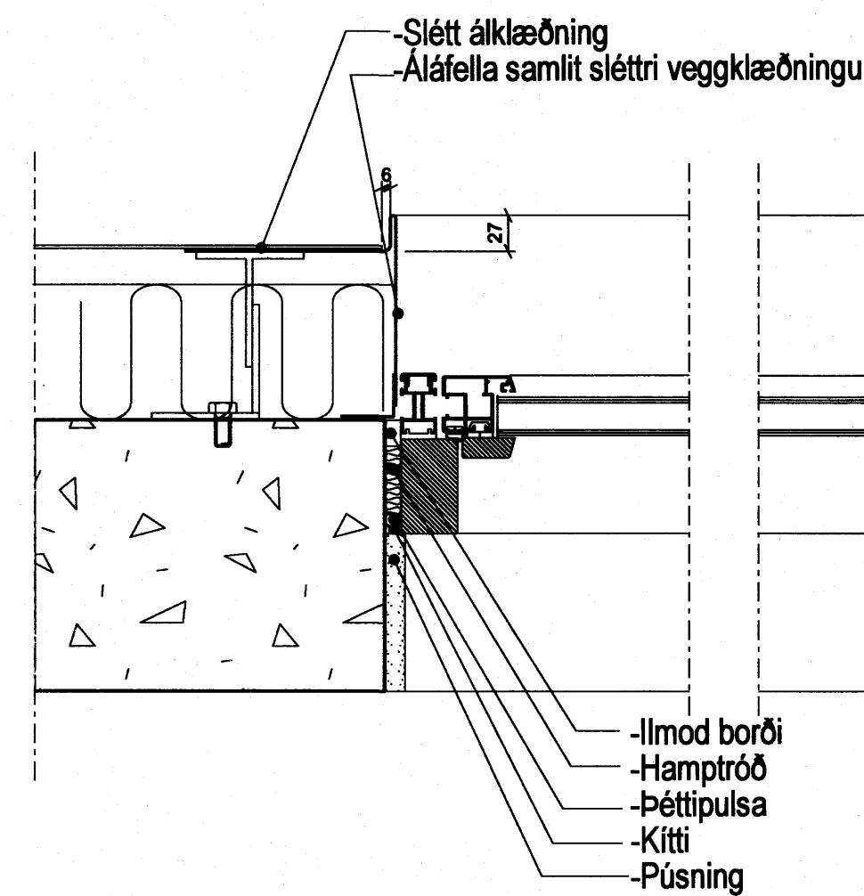
7 DEILI 1:5 Hliðarstykki glugga, slétt álklaðning, efnisskipti við gluggakarm
