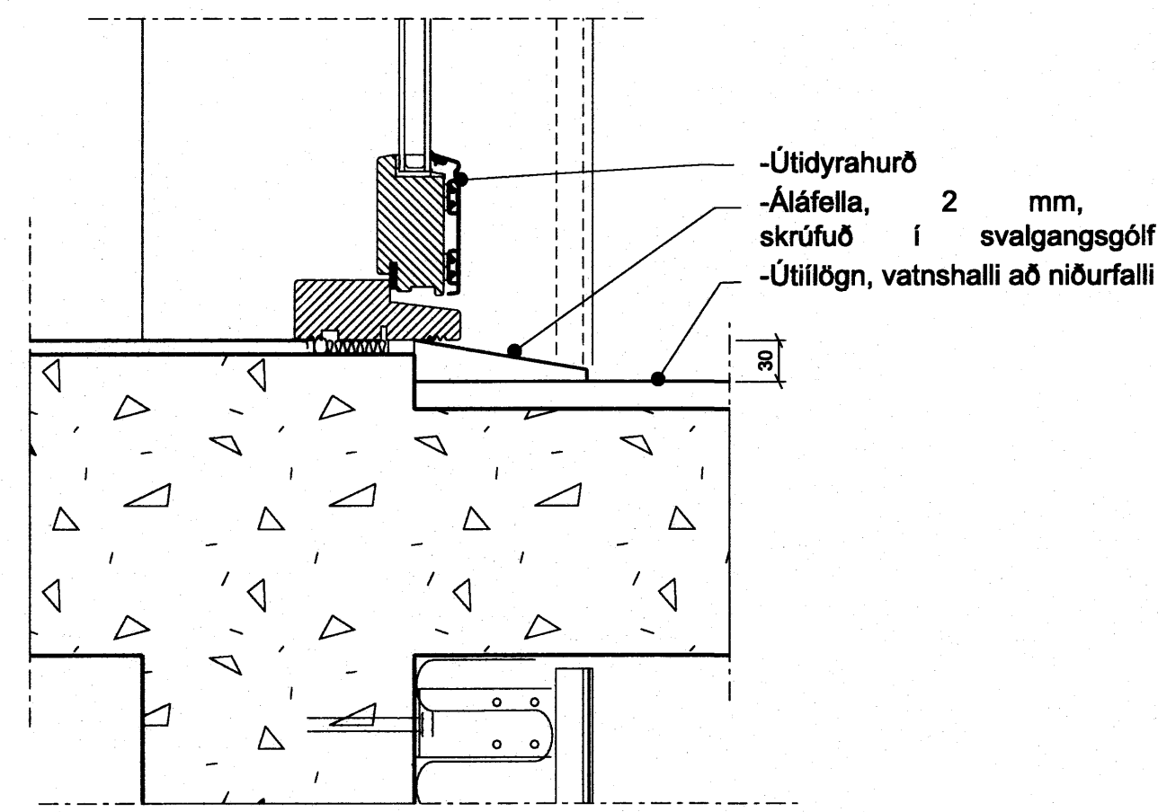
5 DEILI 1:5 Botnstykki útidyrarúða við svalgang
