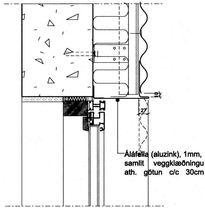
1 DEILI 1:5 Efri brún glugga, báruklæðning
