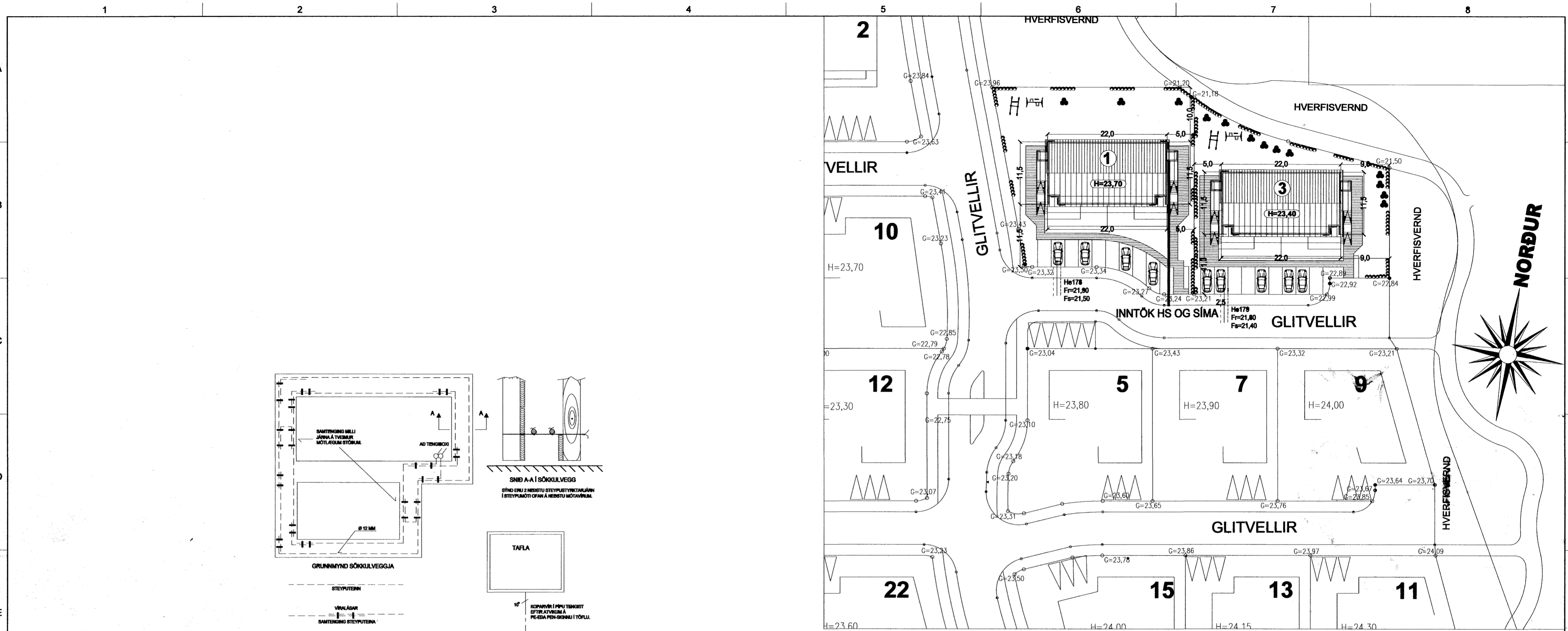
AFSTÖÐUMYND MKV. 1:500
