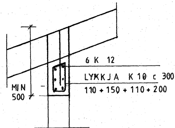
D OG G 1:20
