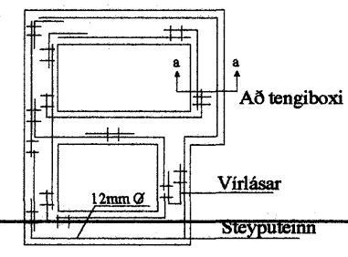
Grunnmynd sökkuleggja
