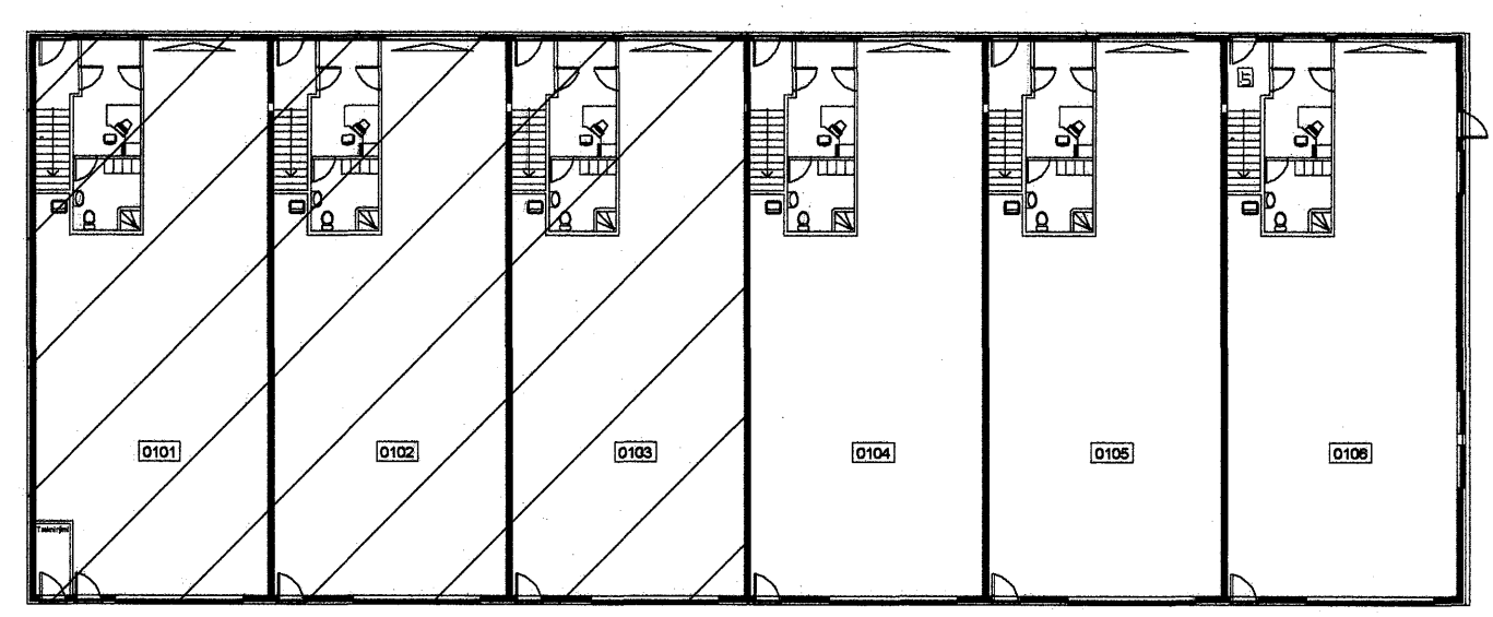
GRUNNMYND 1 HÆÐAR A
