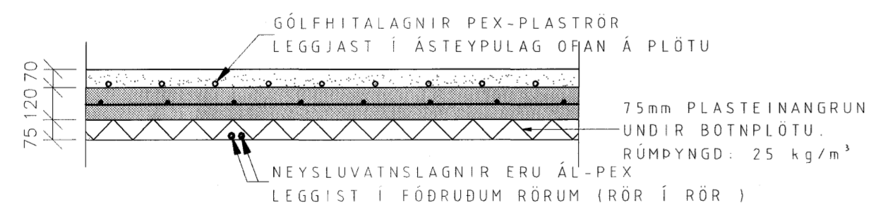
SNIÐ LAGNIR Í BOTNPLÖTU 1:20
