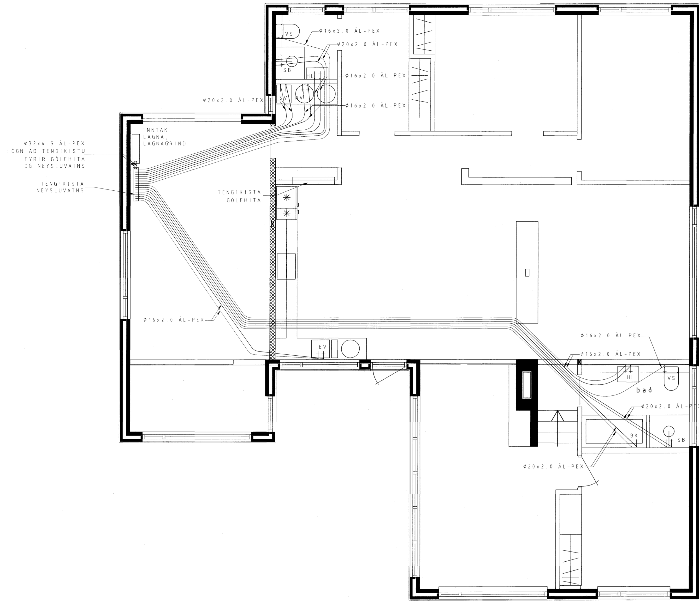
GRUNNMYND NEYSLUVATNS 1:50
