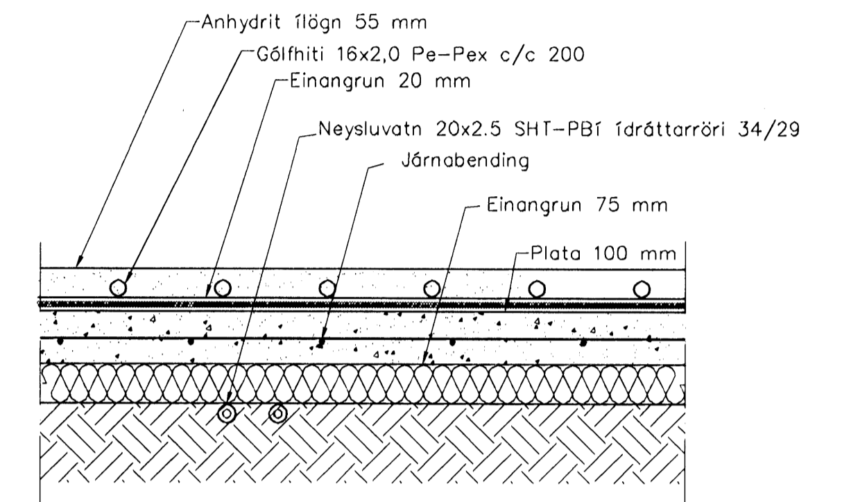
Hita- og vatnslagnir, Sníð í botnplötu, 1:10
