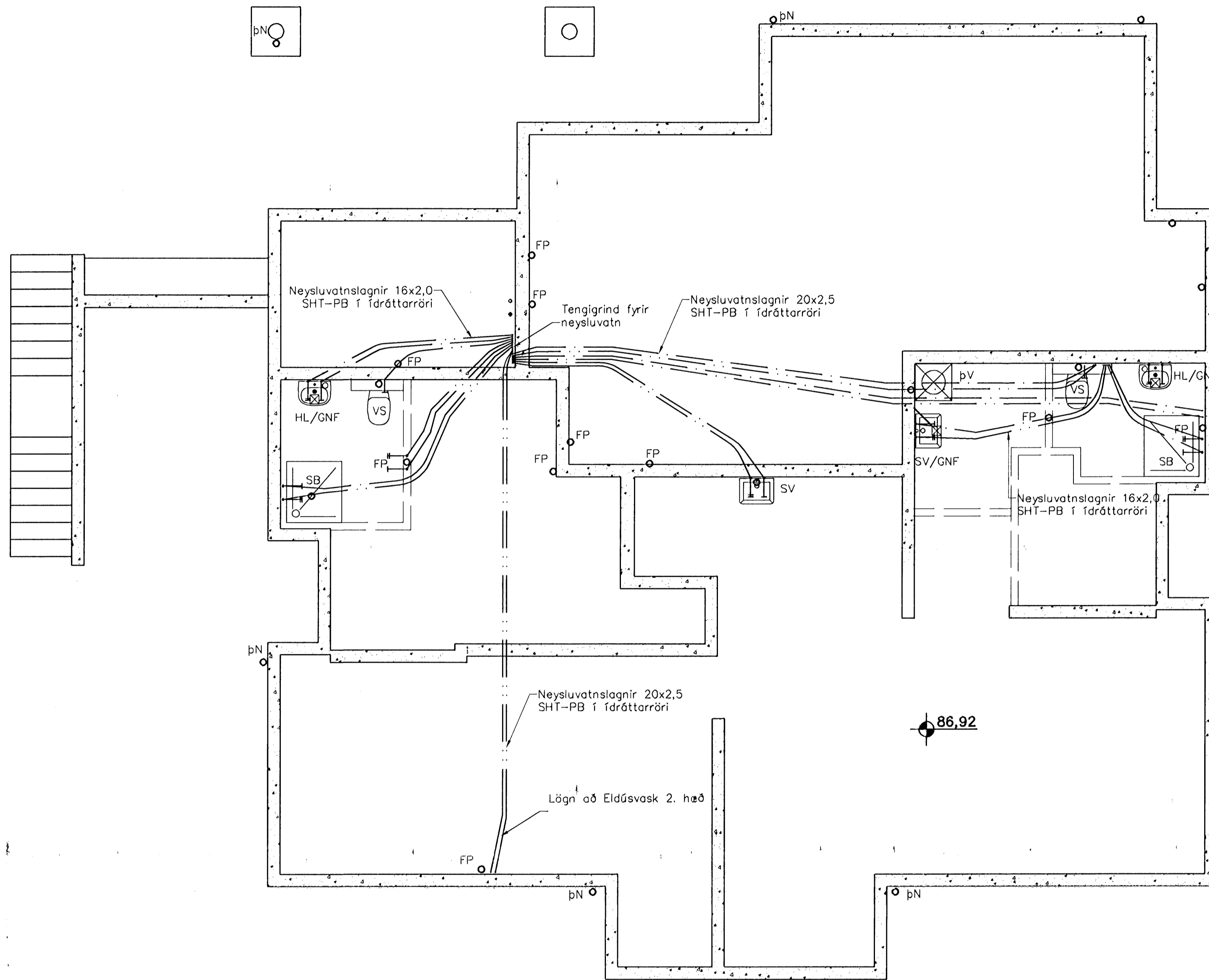
Neysluvatnslagnir 1. hæð, 1:50
