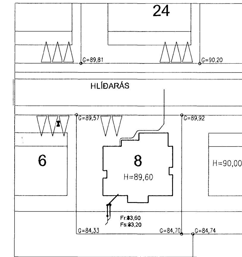
Afstöðumynd 1:50
