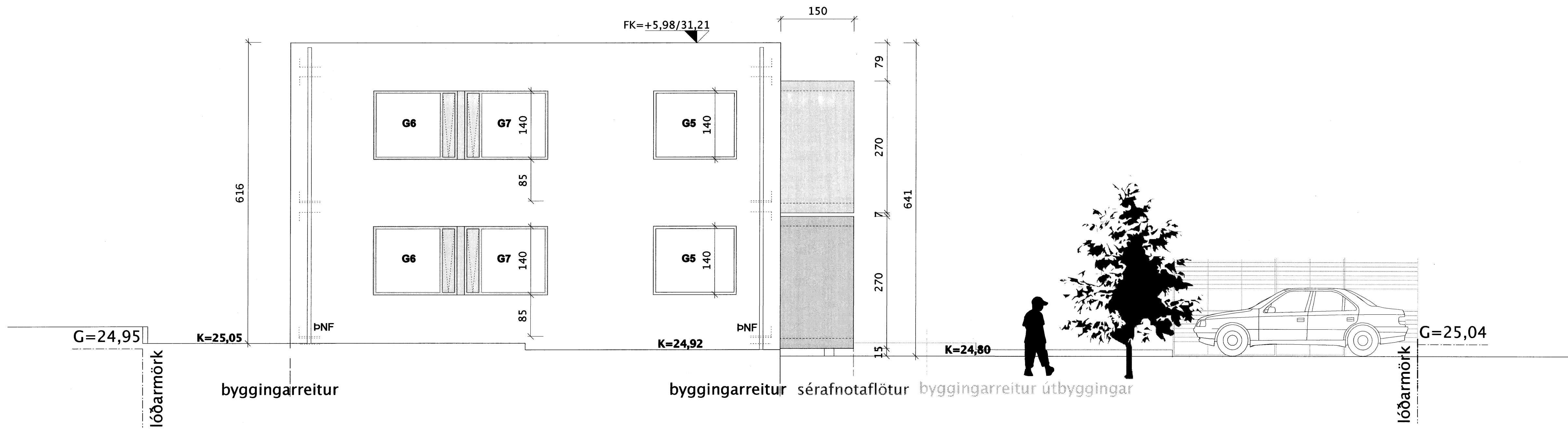
ÚTLIT VESTUR mkv. 1:100
