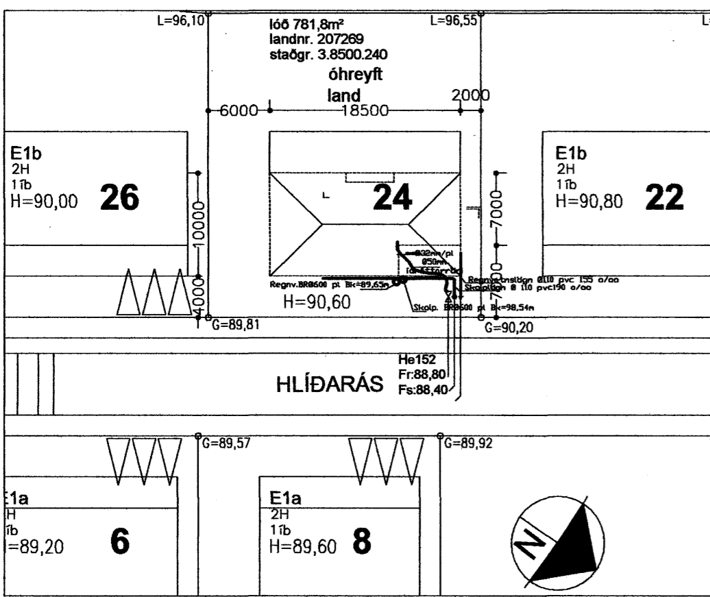
Afstöðumynd Mkv 1:500
