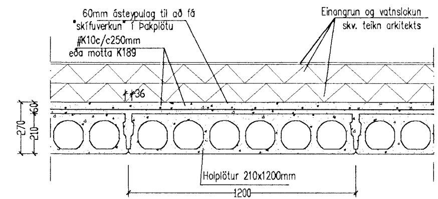
Snið P8 1:20 Almennt snið í þakplötu/holplötu Holplötu 210x1200mm
