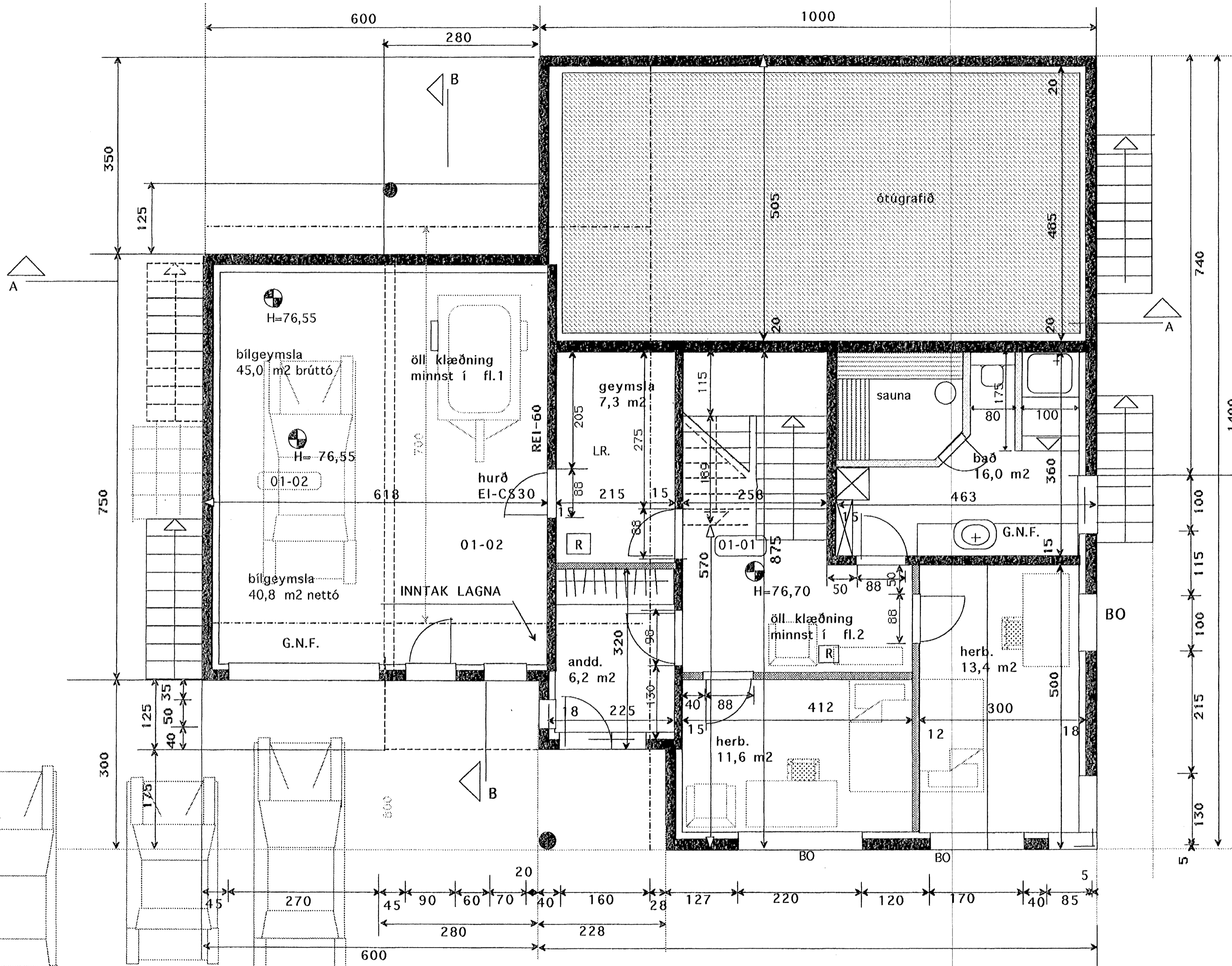
GRUNNMYND 1:50
