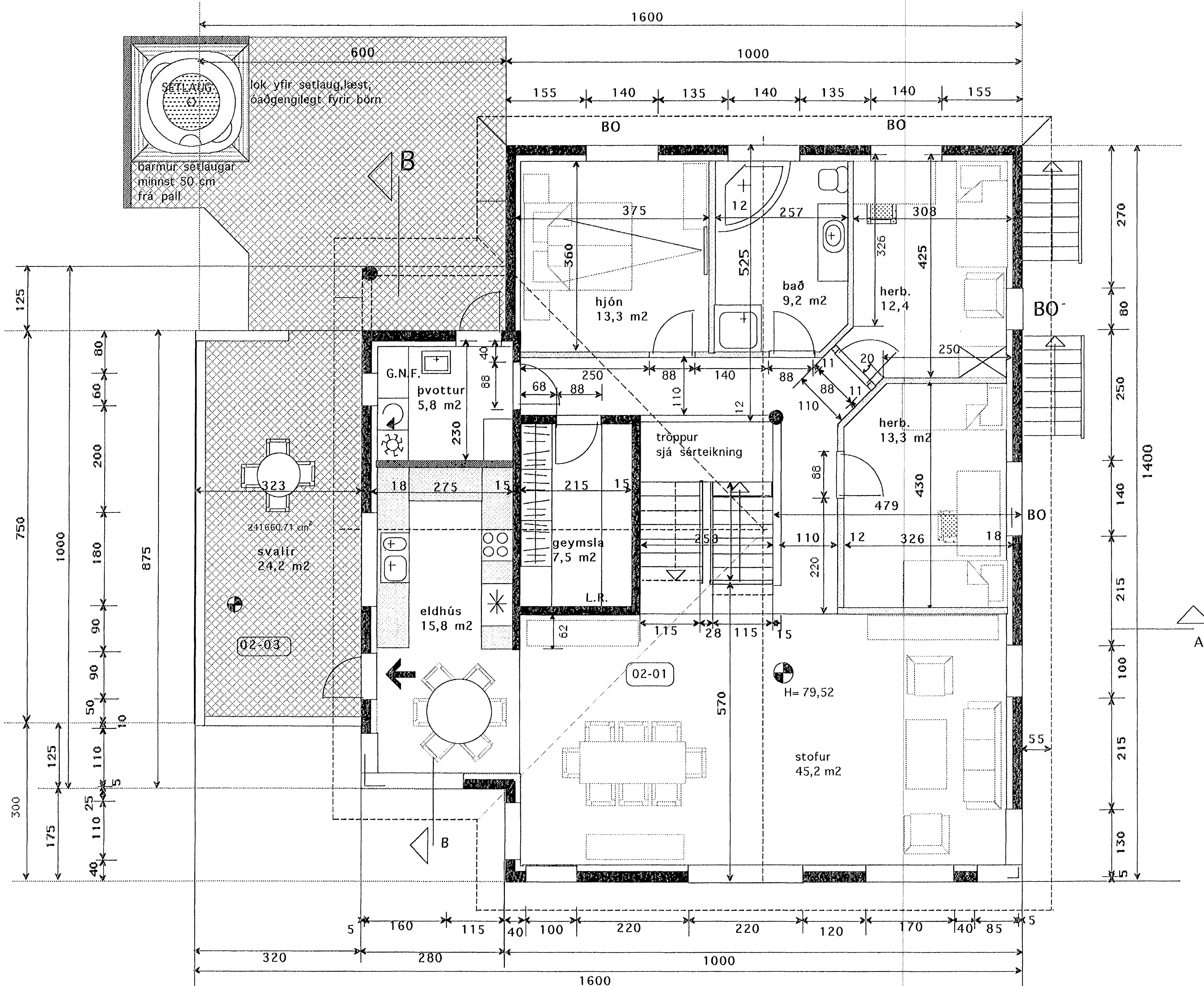
GRUNNMYND 2 HÆÐ 1:50
