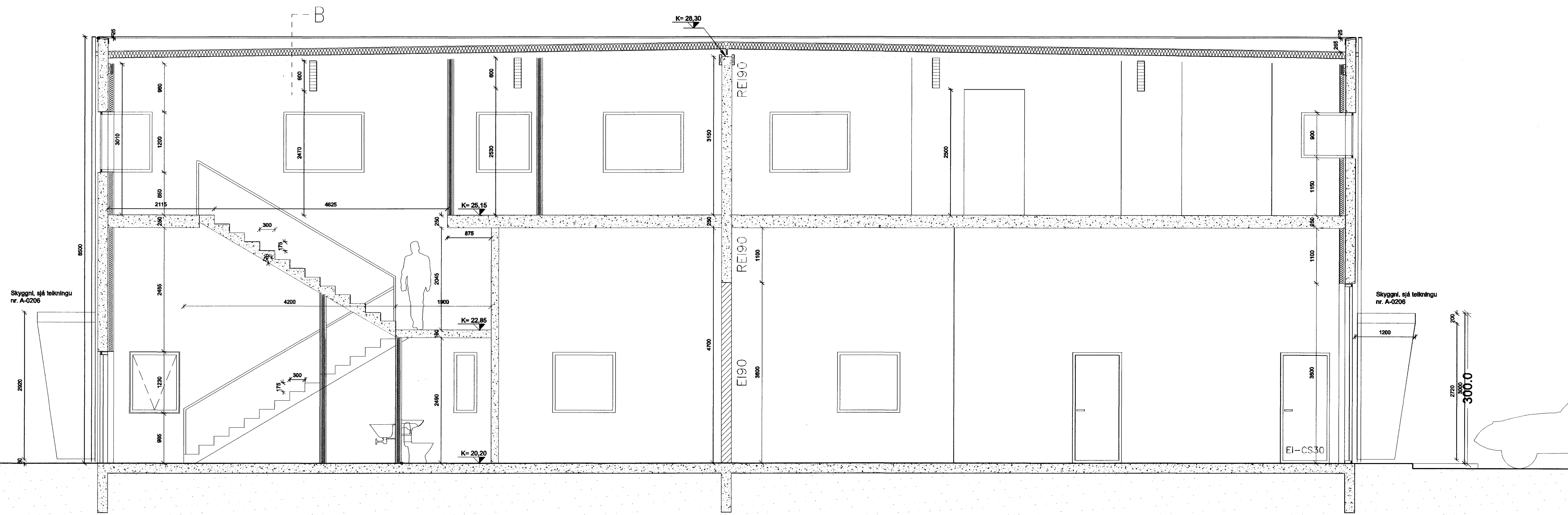
SNID A-A 1:50
