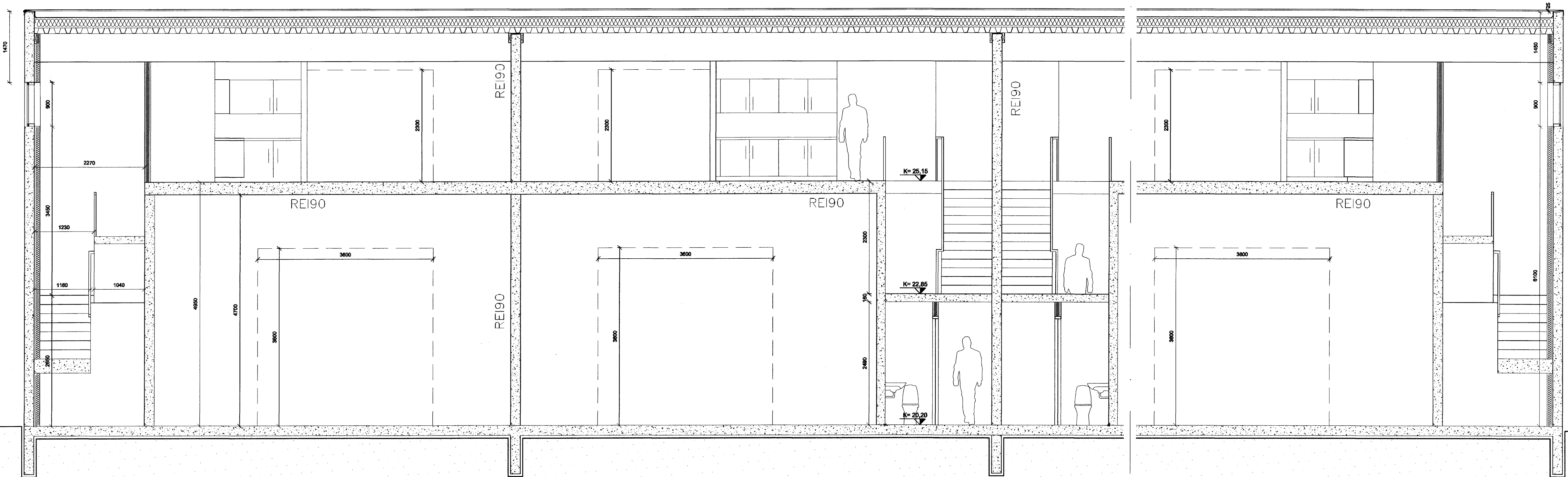
SNID B-B 1:50
