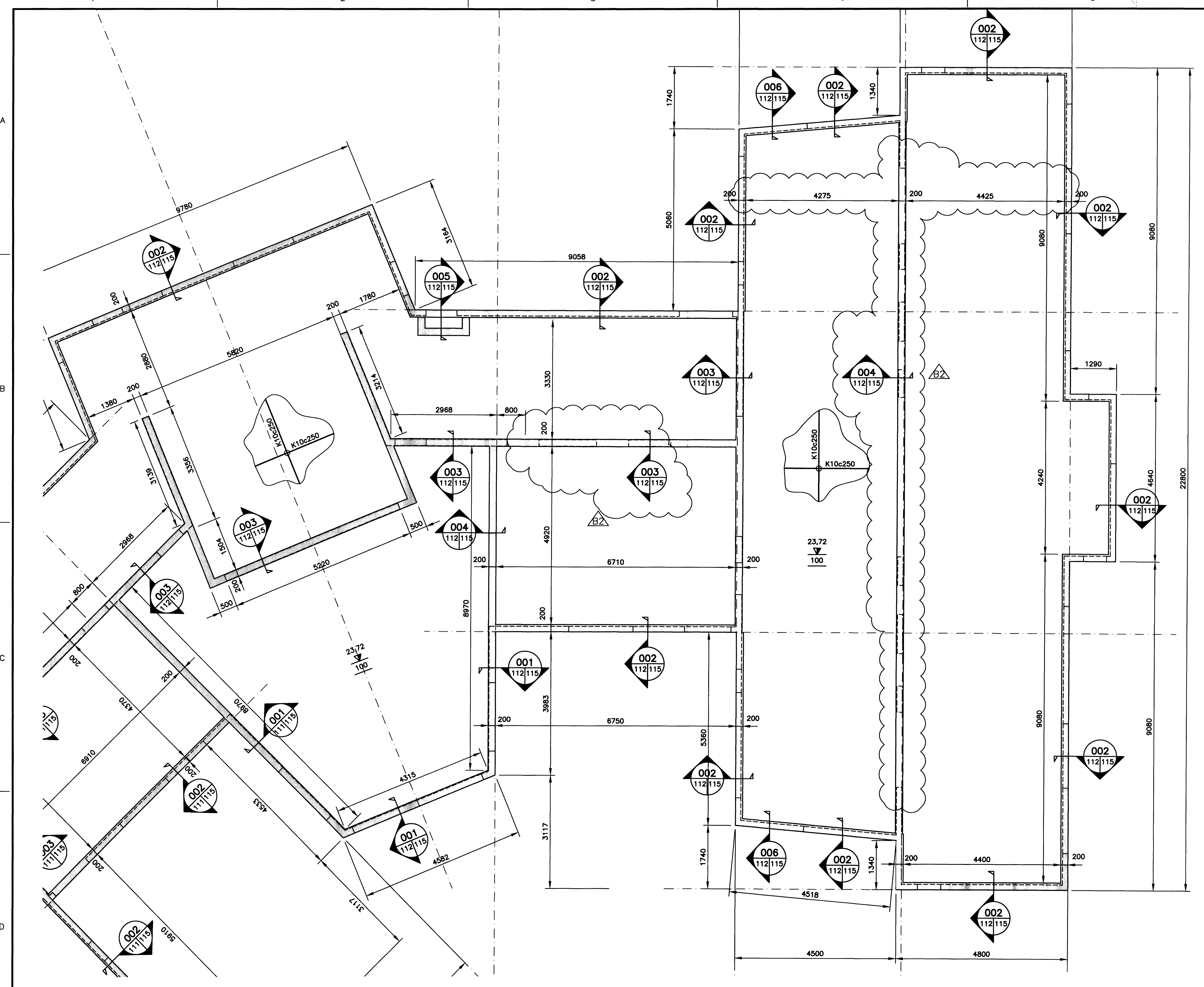
UNDIRSTÖÐUR. GRUNNMYND MKV. 1
