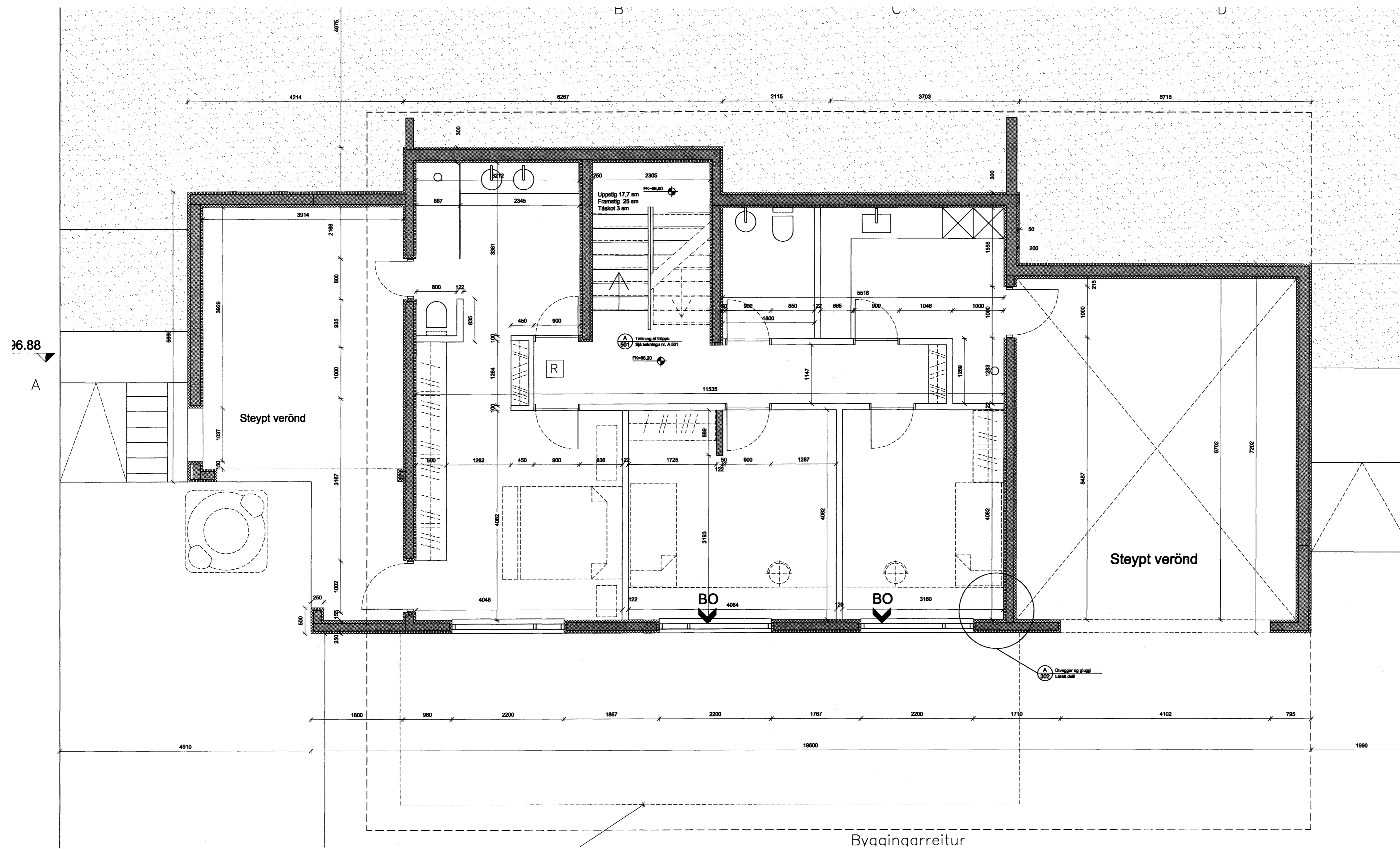
GRUNNMYND NEDRI HÆÐAR, 1:100
