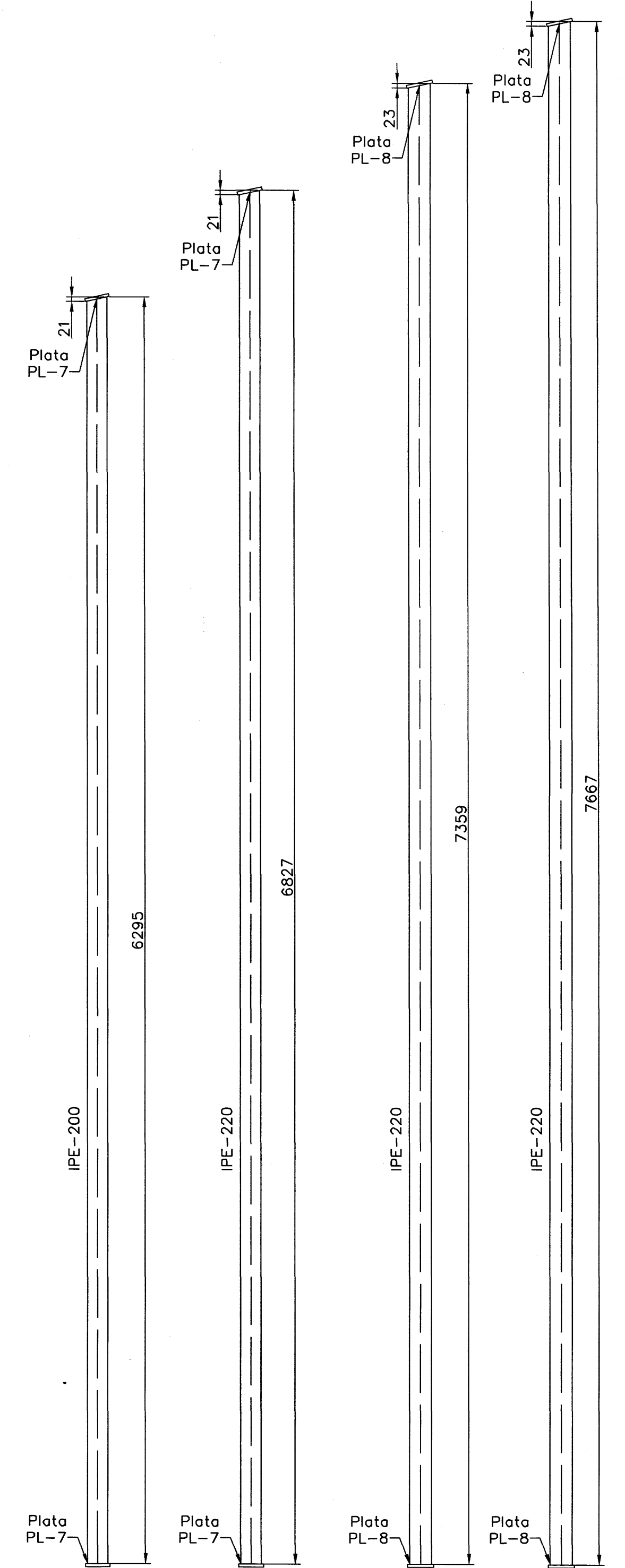
Gafflstoðir 2 stk. 1:20
