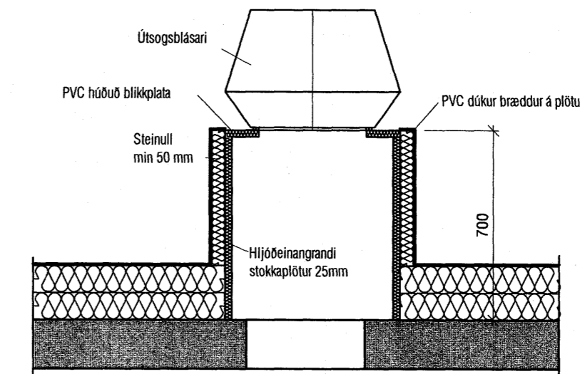
Sníð í safnkassa og stökk á þaki
