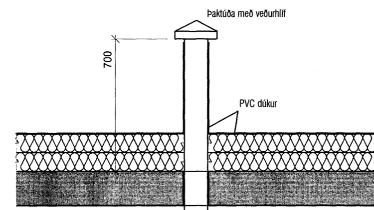
Sníð í lofttöðu fyrir stigahús 1:20
