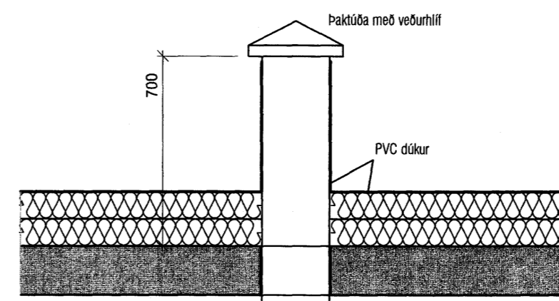
Sníð í lofttöðu fyrir lyftustökk 1:20
