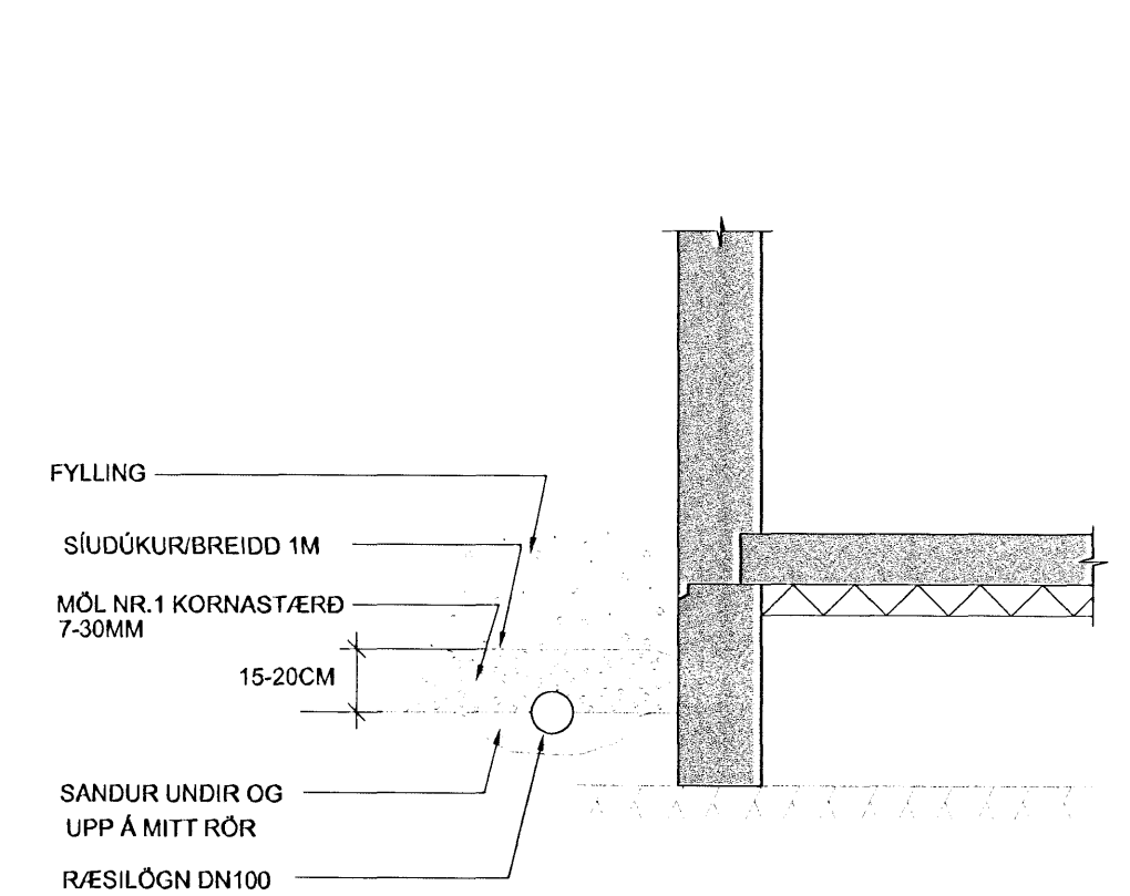
SM4 RÆSILÖGN, 1:20 DÆMIGERT ÞVERSNIÐ
