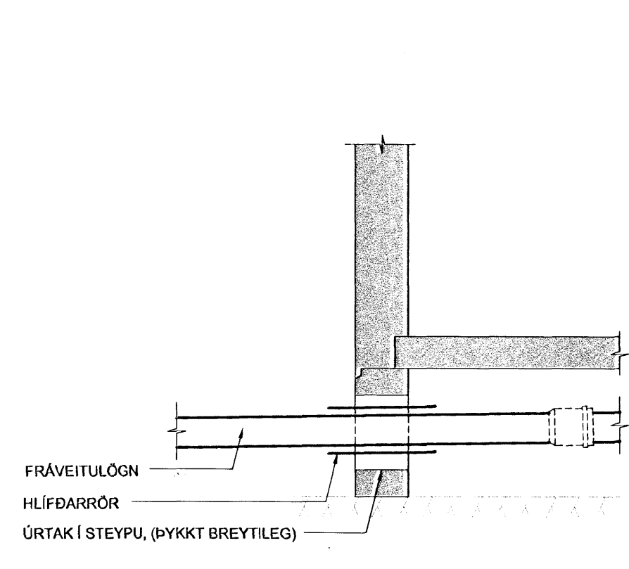
SM3 LÖGN GEGNUM UNDIRSTÖÐU, 1:20 DÆMIGERT ÞVERSNIÐ
