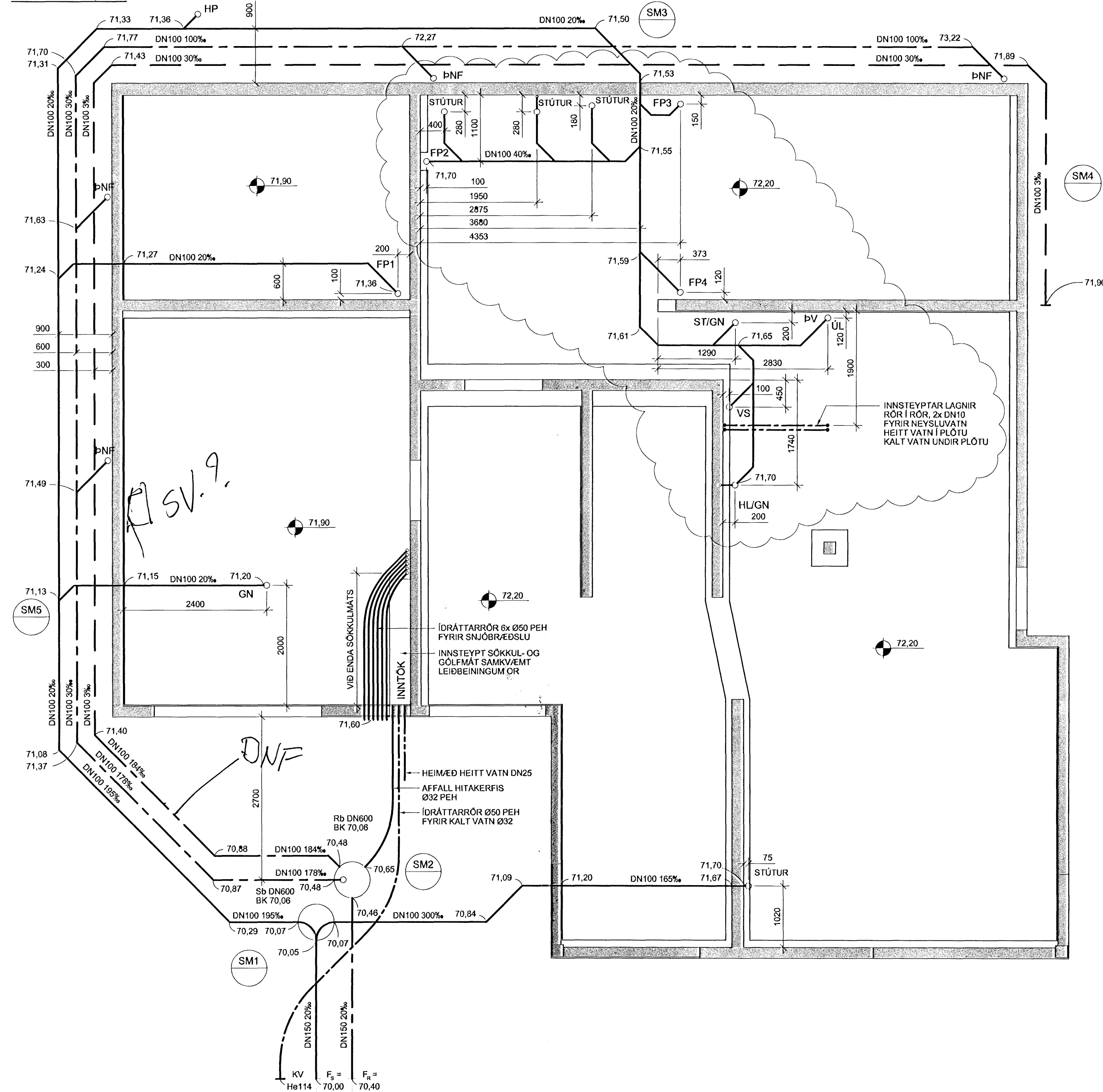
GRUNNMYND, 1:50
