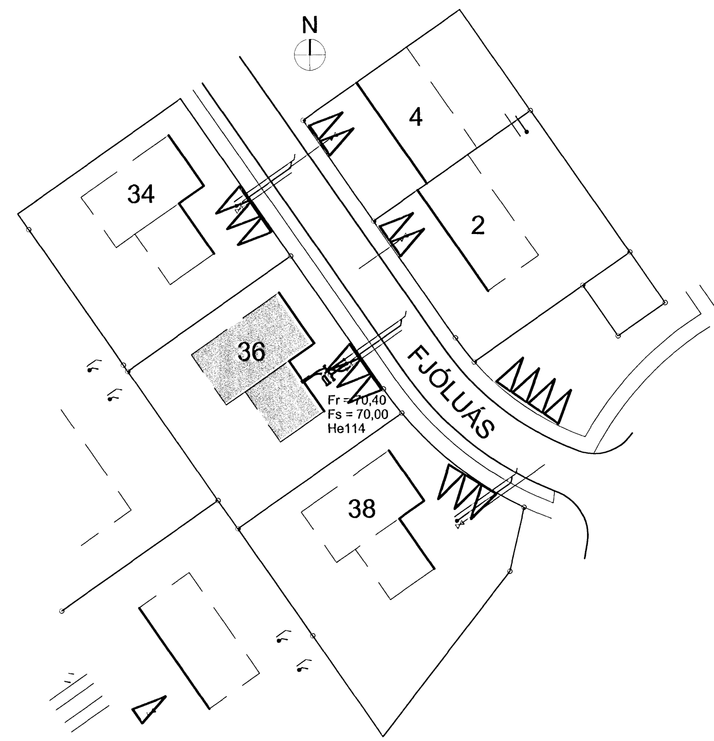
AFSTÖÐUMYND, 1:500
