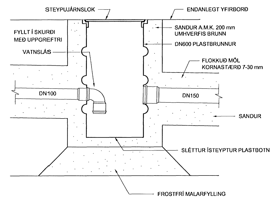
SM2 DN600 REGNVATNSBRUNNUR, 1:20 DÆMIGERT ÞVERSNIÐ
