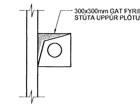
SM6 GÖT Í PLÖTU, 1:20
