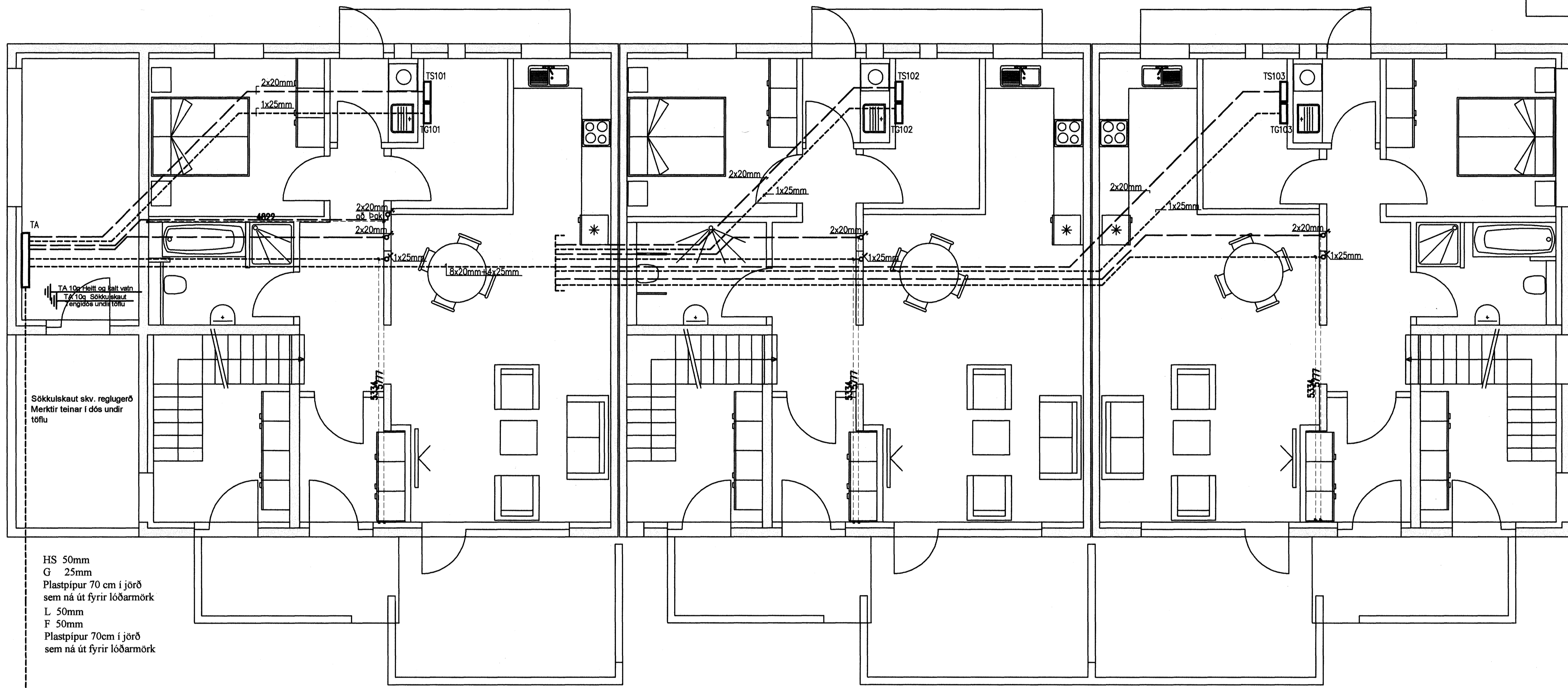
Inntök, hvíslar og töflur mkv. 1:50
