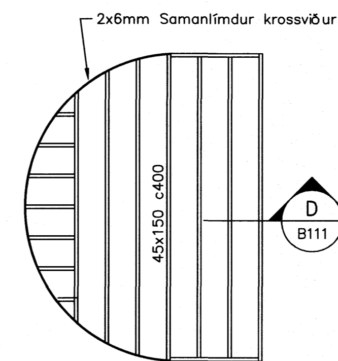
— Grunnmynd — Efra gólf — 1:50
