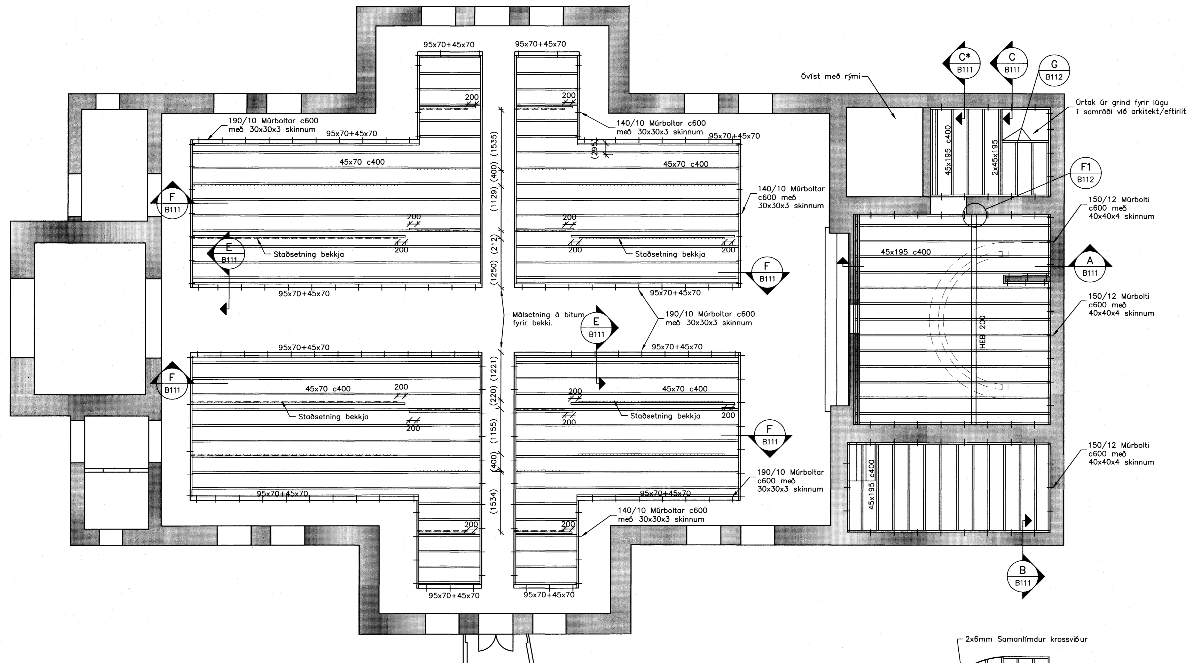
— Grunnmynd 1. hæðar — Bitar — 1:50
