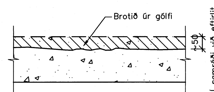
— Kennisnið — Máluð gólf — 1:10
