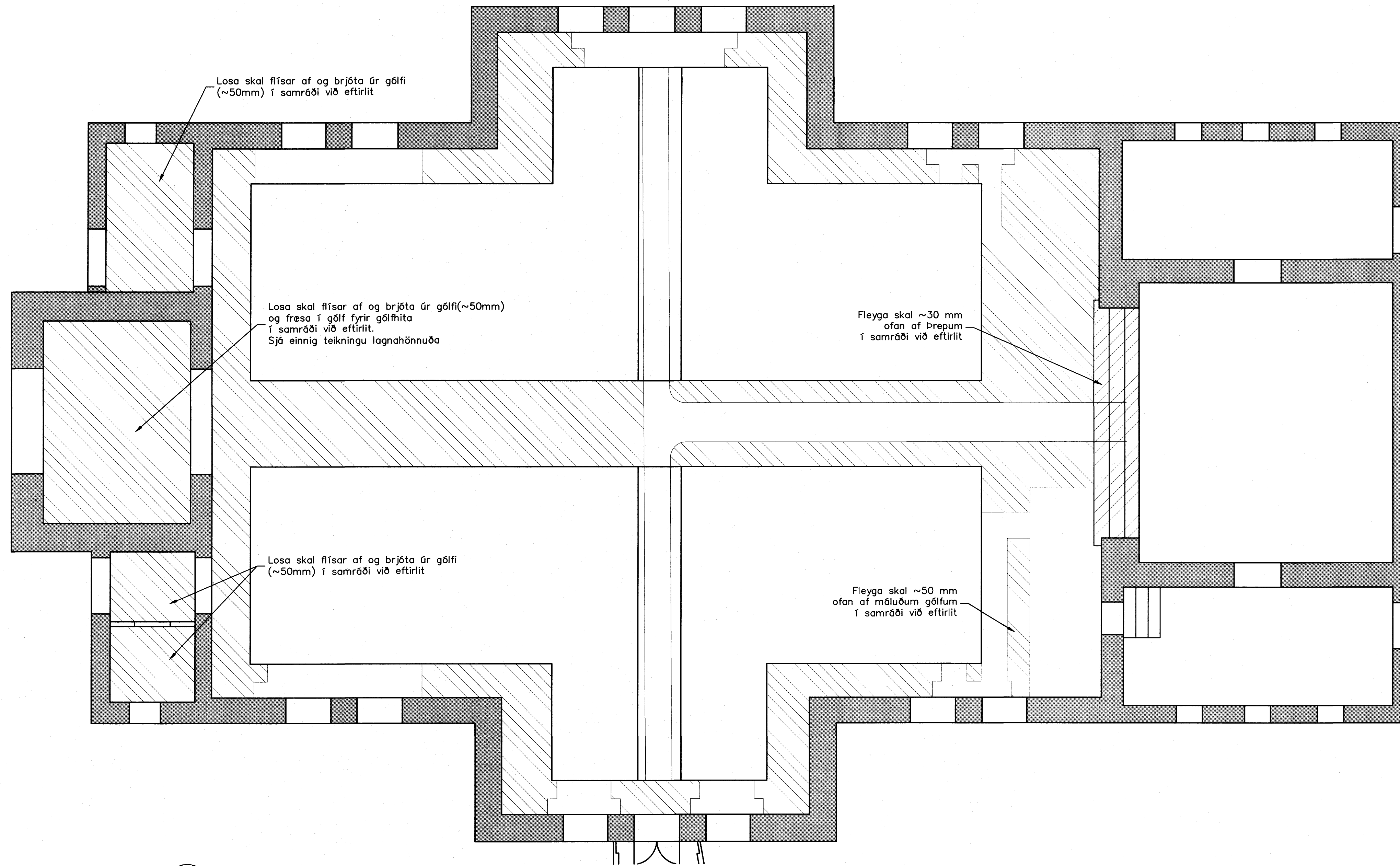
— Grunnmynd — Fleygun úr gólfi — 1:50
