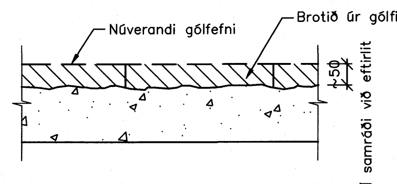
— Kennisnið — Flísalögð gólf — 1:10
