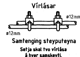
Tengja skal saman tvö neðstu járnin í sökkulveggjum allan úthringinn og að upptaki í tengibox. Í raðhúsum, þarhúsum og hlöðstæðum húsum er leyfing að tengja samantenging úthring, en tengibox og tenging verðr við hverja heiltöng.
