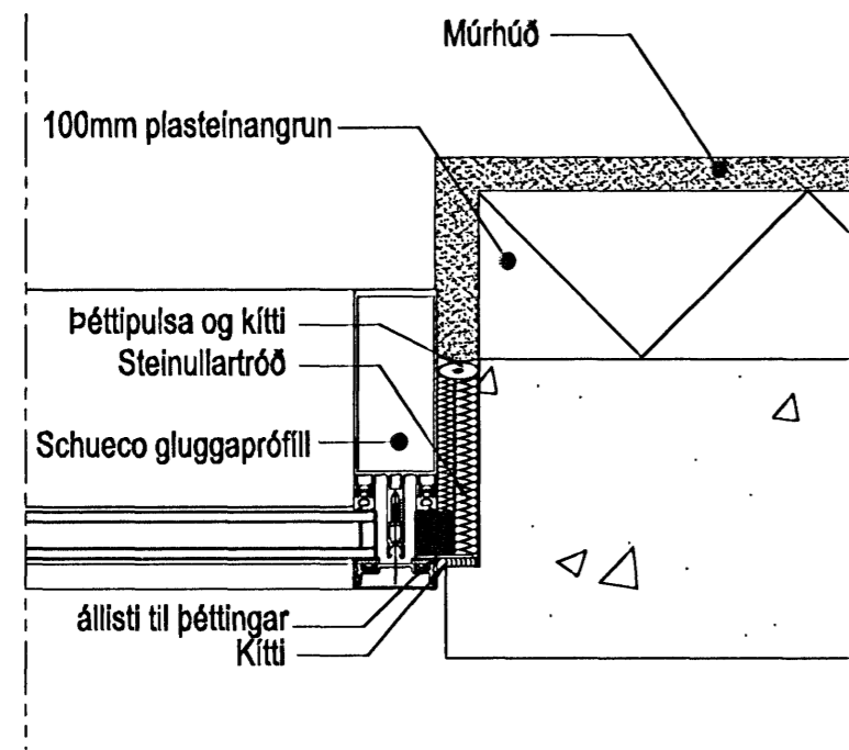
Frágangur 120mm glugga - lárétt snið
