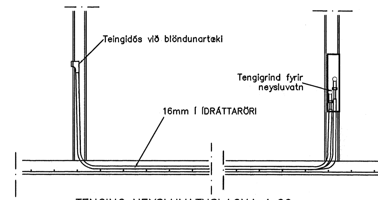
TENGING NEYSLUVATNSLAGNA 1:20
