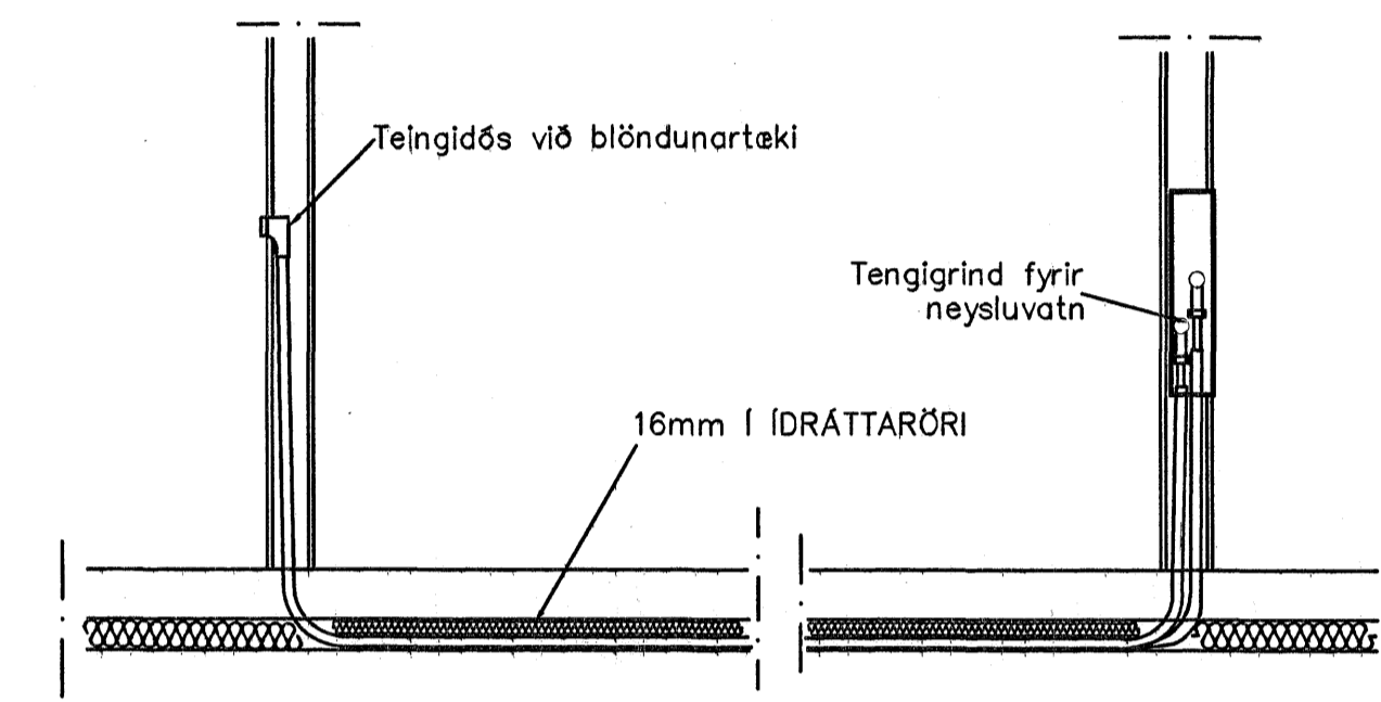
TENGING NEYSLUVATNSLAGNA 1:20
