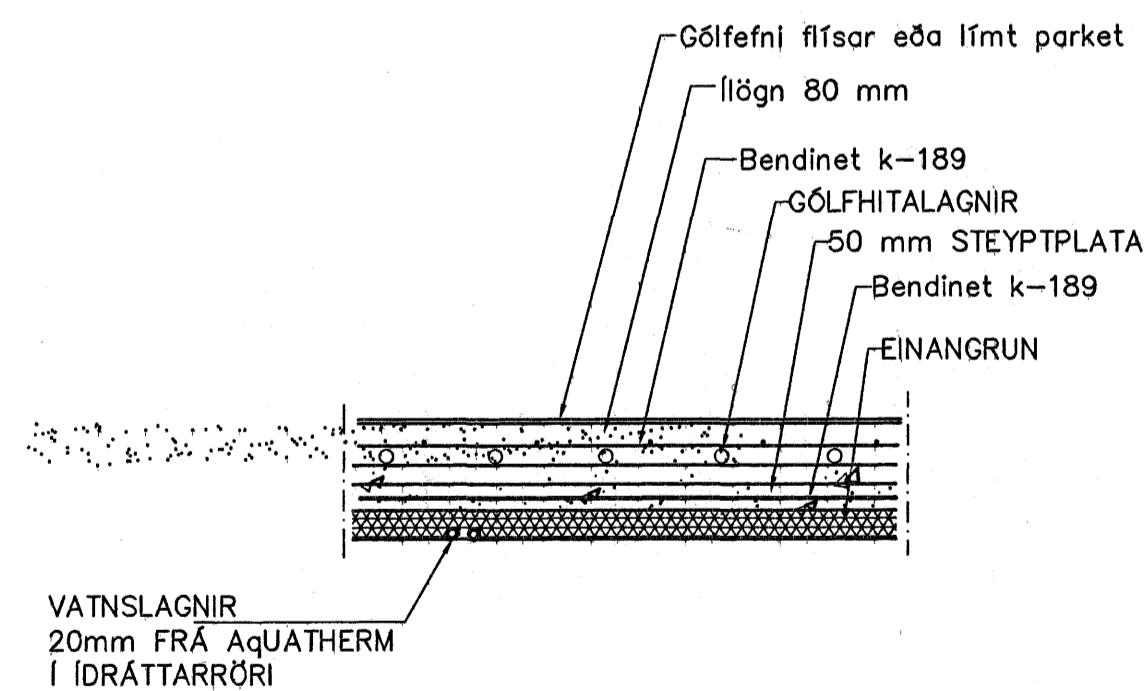
LAGNIR, SNIÐ, 1:20
