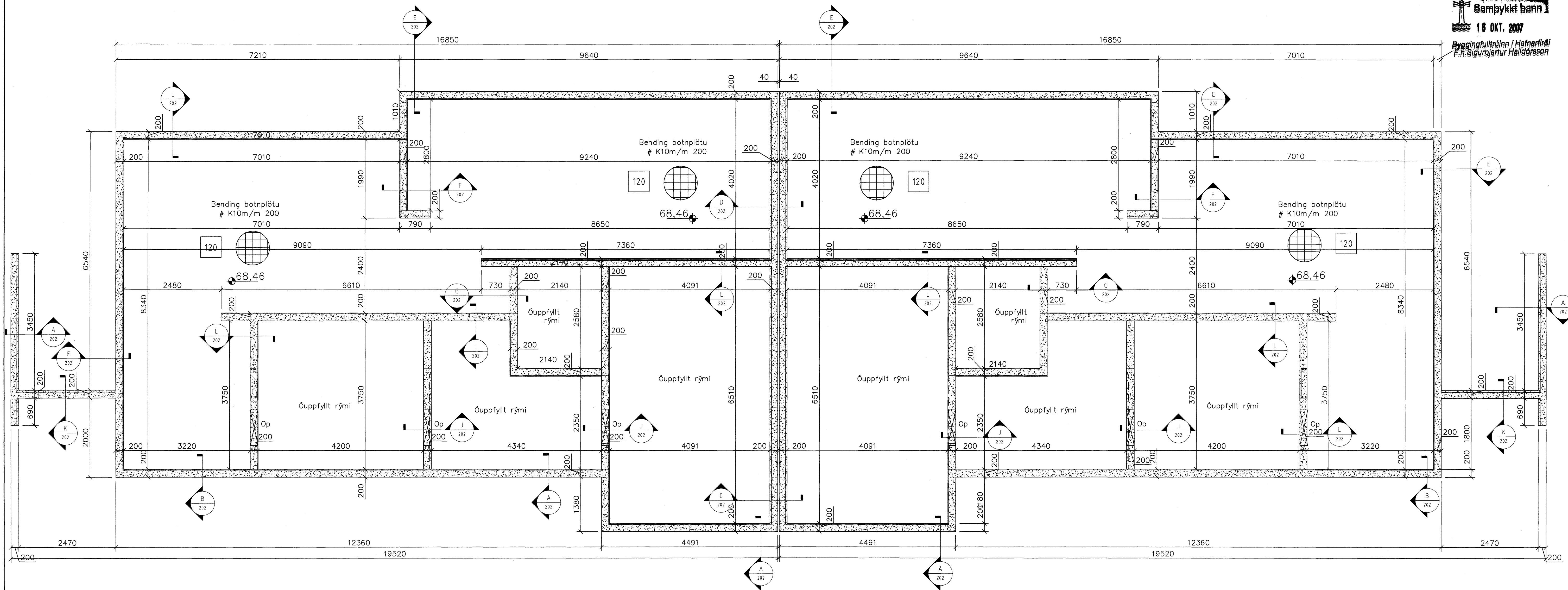
Grunnmynd neðri hæðar 1 = 50 mm
