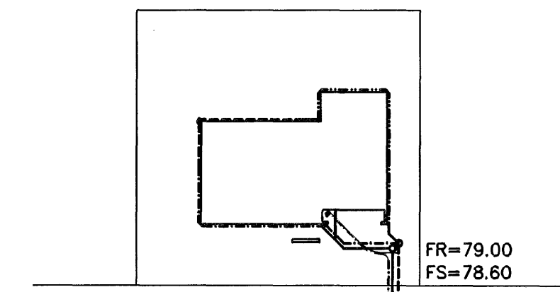
AFSTÖÐUMYND 1:50
