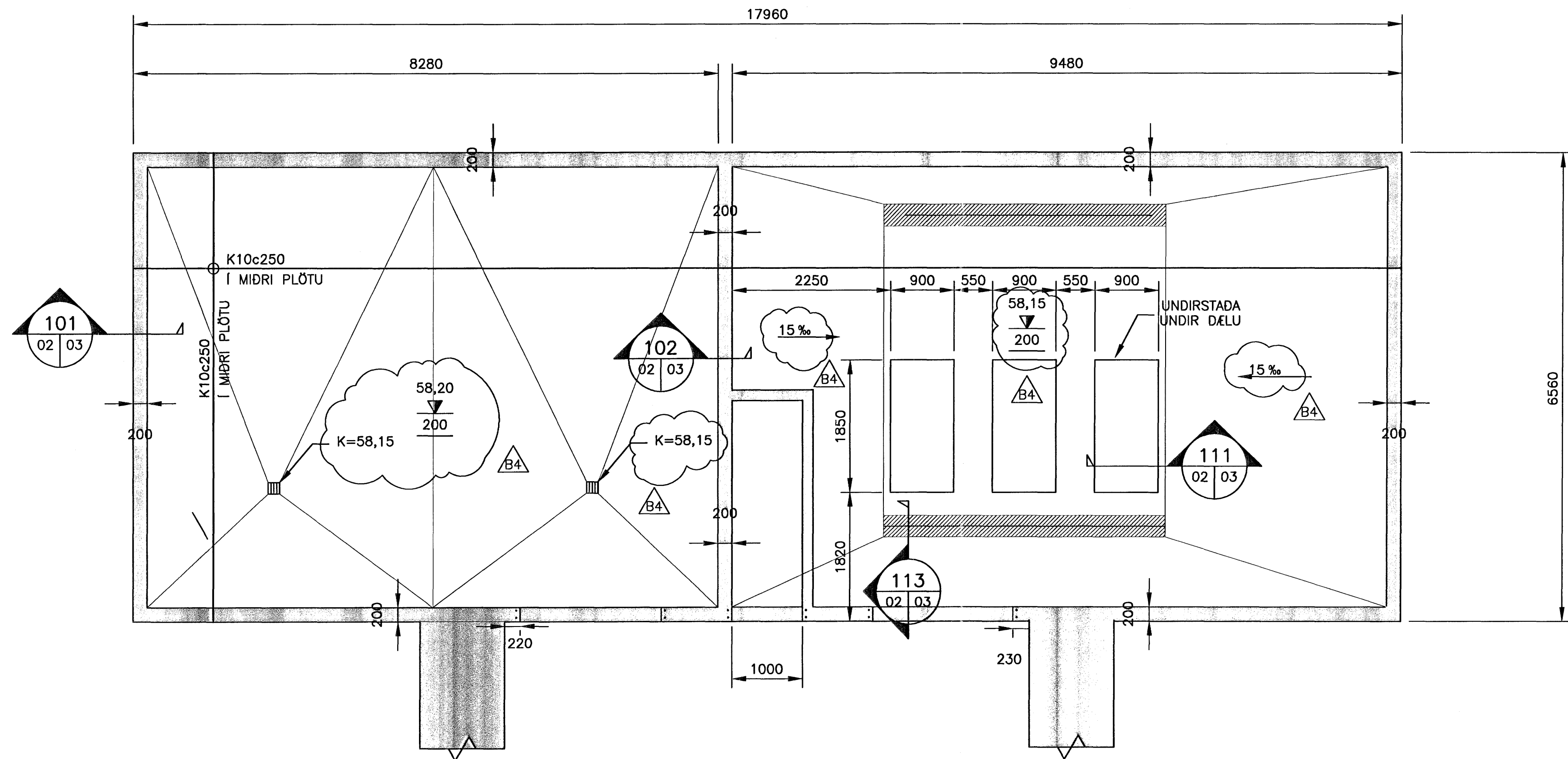
GRUNNMYND, UNDIRSTÖÐUR OG BOTNPLATA 1:50
